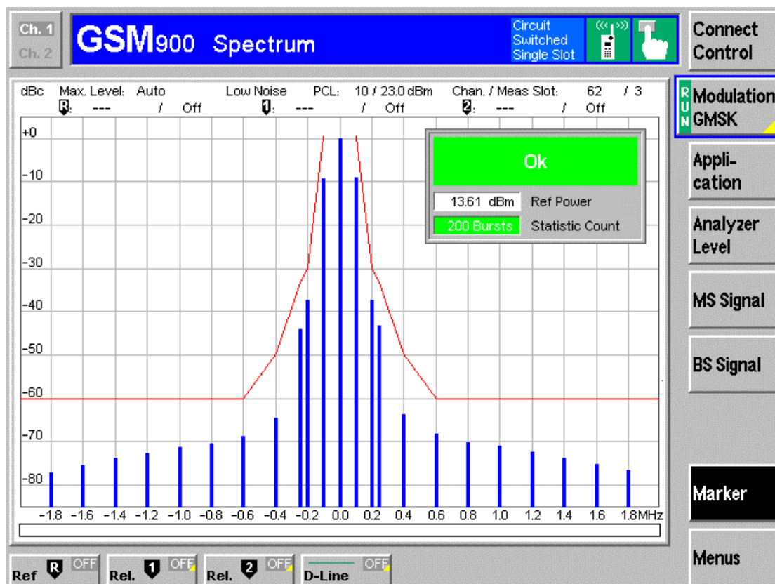
图 2—48 GSM900 Spectrum_Marker_ Modulation GSMK
