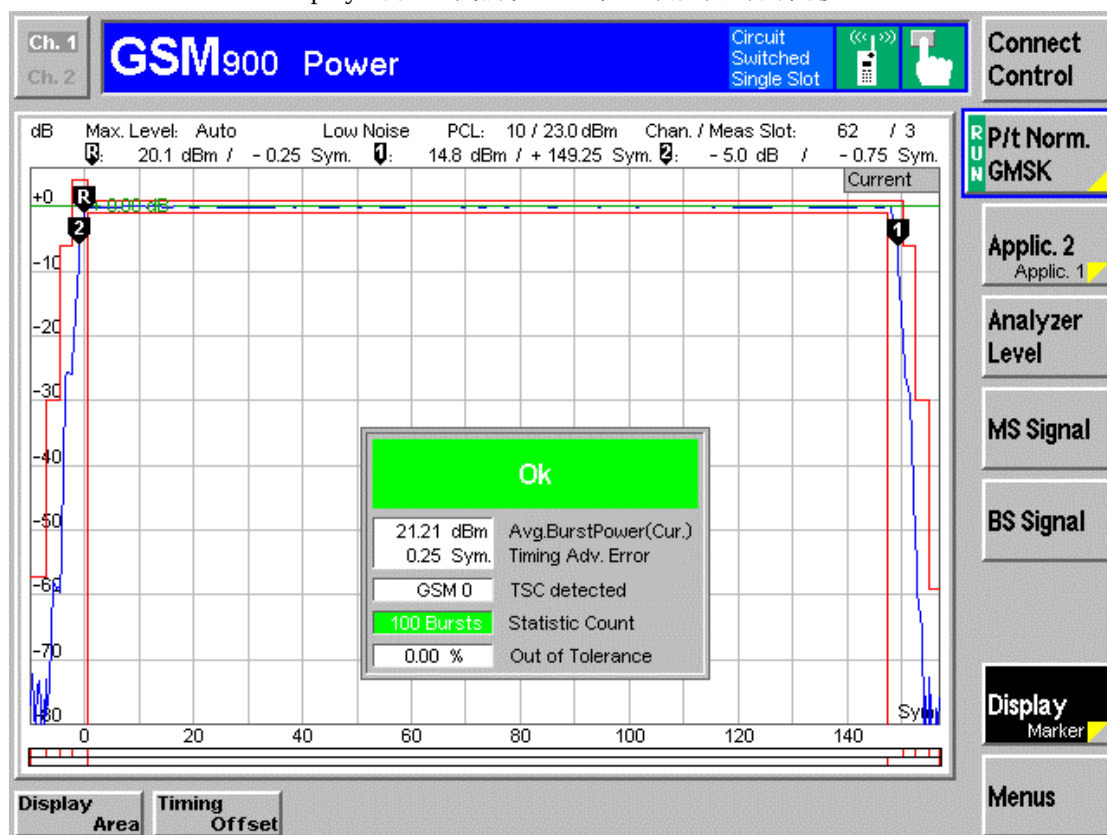
图 2—30 GSM900 Power_Display
