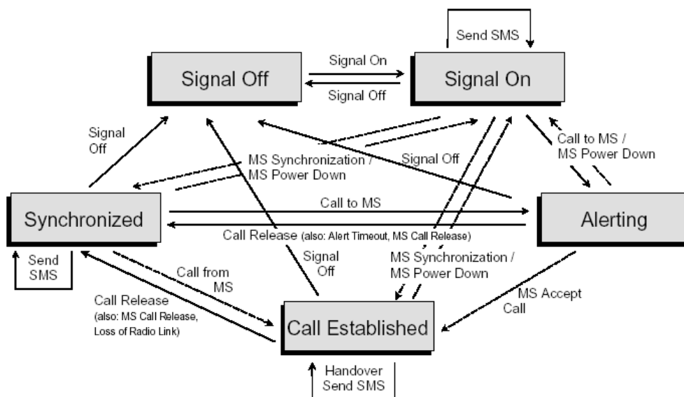
图 2-1 CMU200 信令测试模式下的状态转换。
