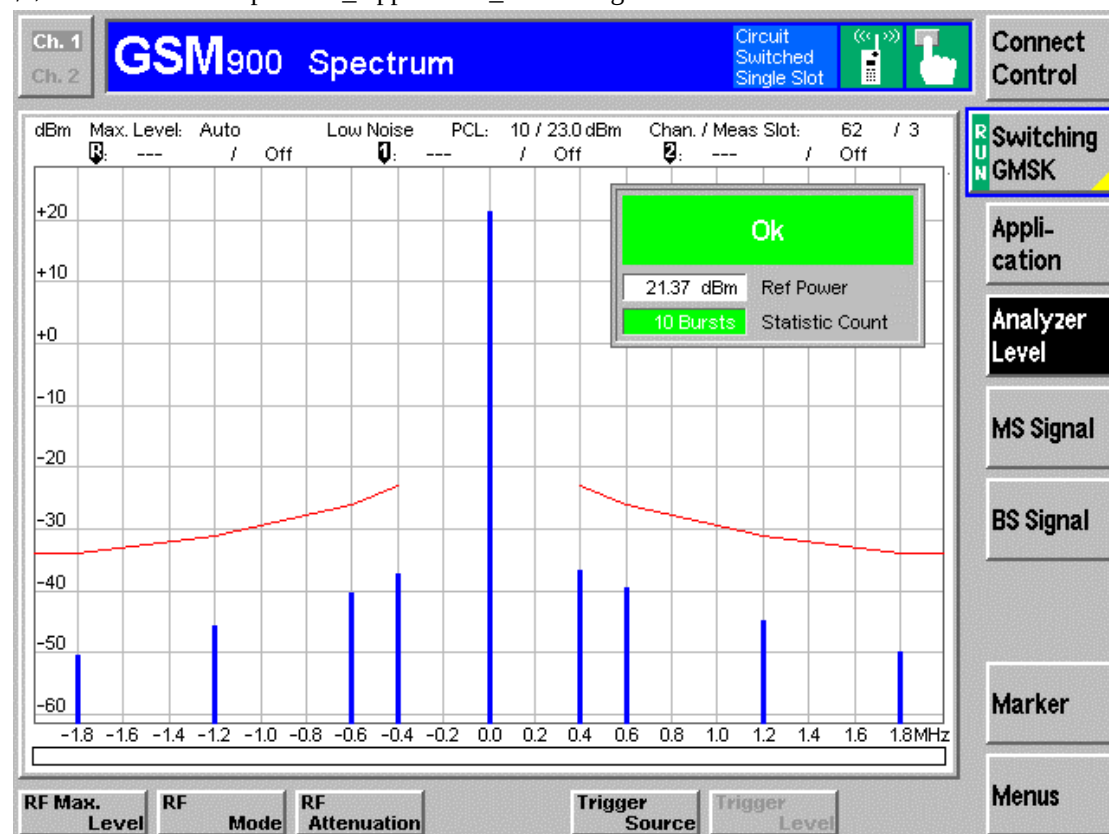
图 2—49 GSM900 Spectrum_Application_ Switching GMSK
