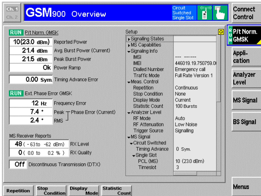
图 2—15 GSM 900 Overview_P/t Norm.GMSK
