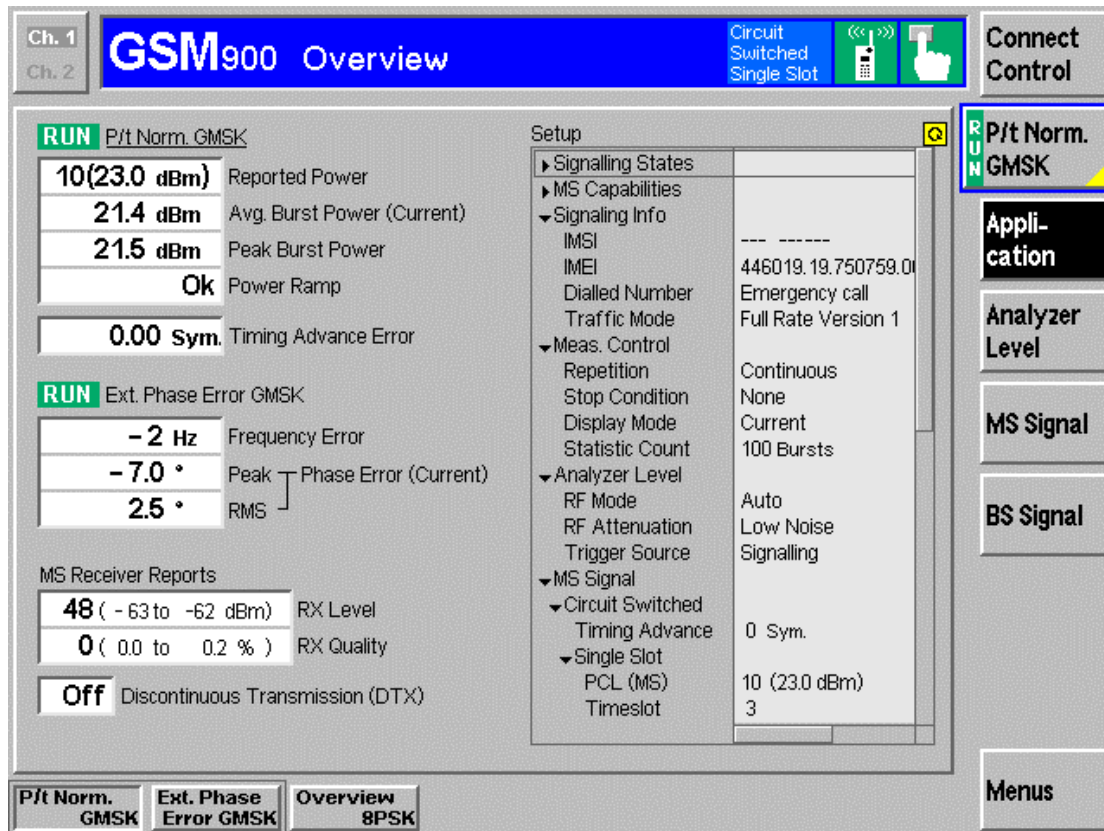
图 2—16 GSM 900 Overview_Application
