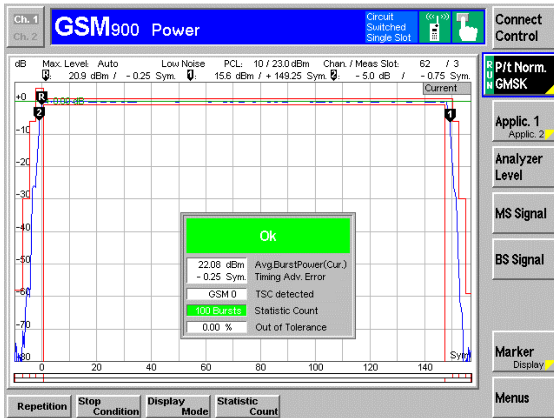
图 2—21 GSM900 Power_P/t Norm. GMSK
