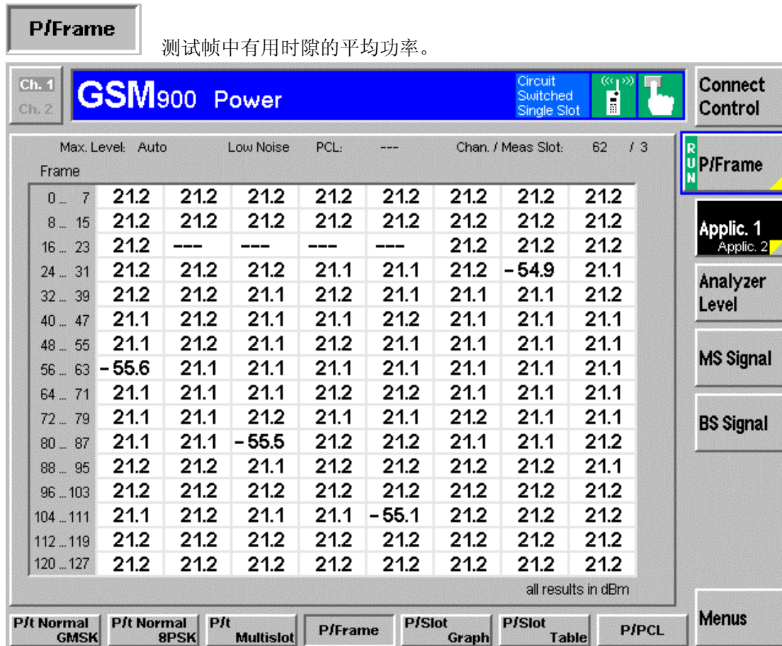
图 2—15 GSM900 Power_Applic.1_ P/Frame
