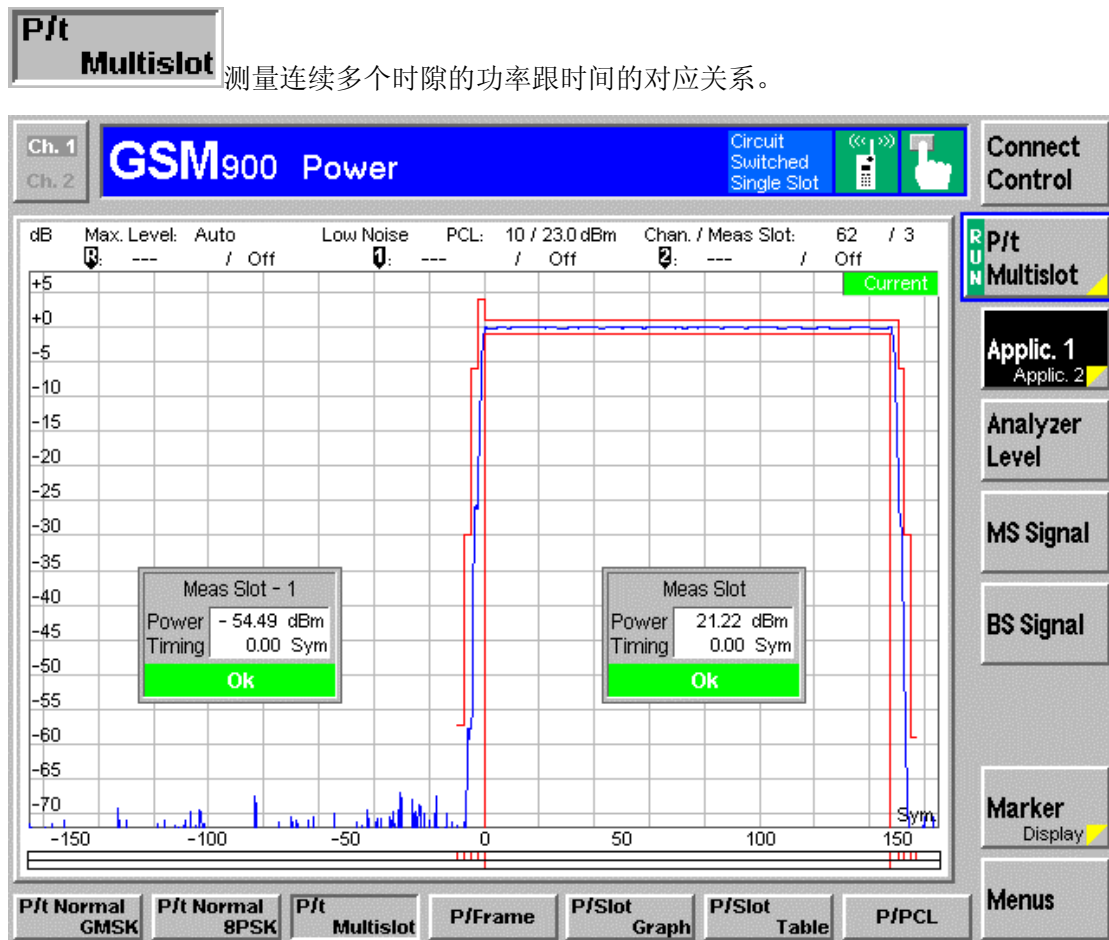
图 2—24 GSM900 Power_Applic.1_ P/t Multislot
