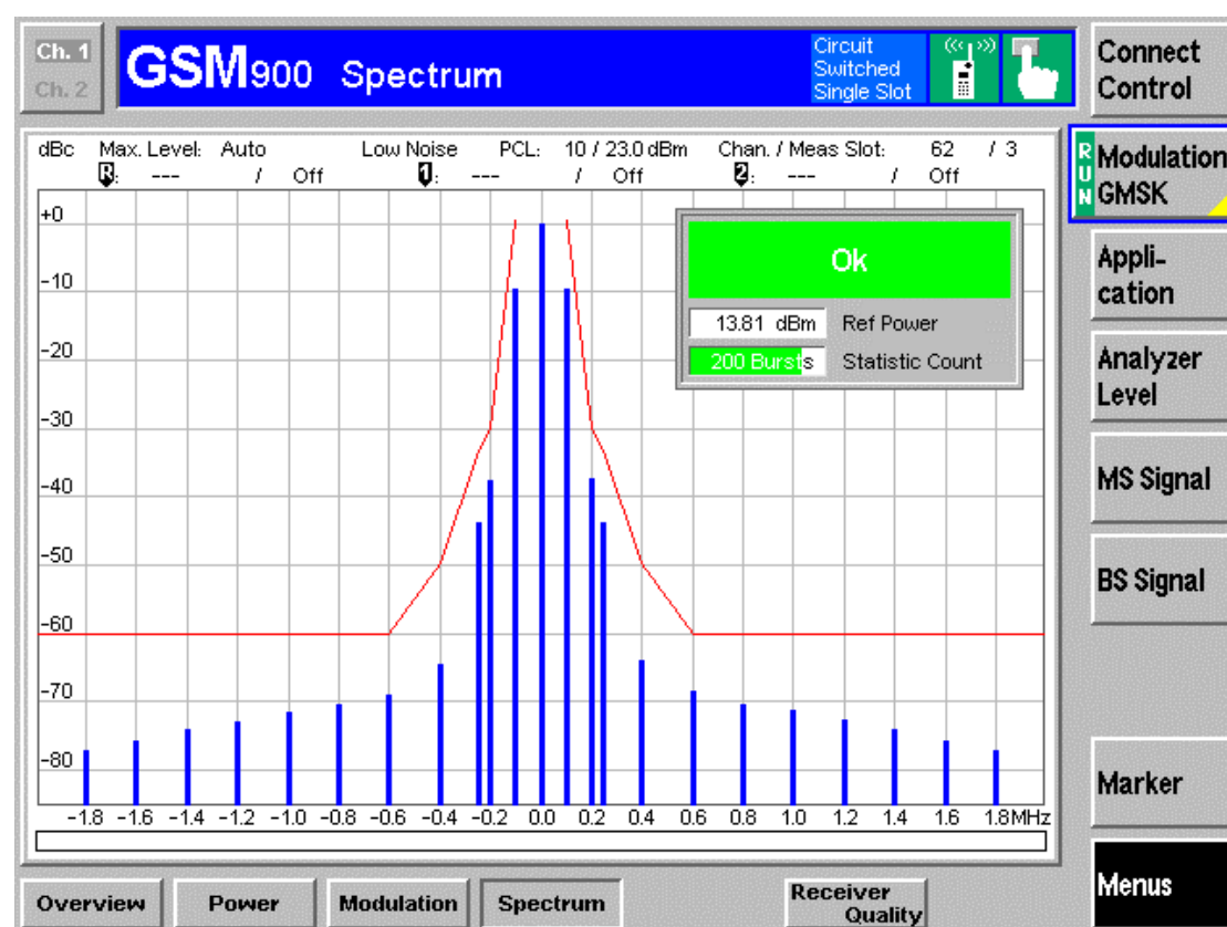
图 2—43 GSM900 Spectrum
