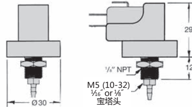
0.187 (4.75) 快速接头
