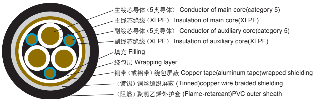
3+3芯 BPYJVP12R、ZR-BPYJVP12R BPYJVPX13R、ZR-BPYJVPX13R
