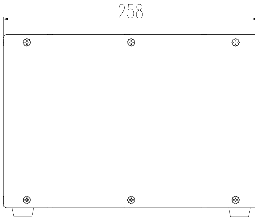
图 2 产品侧视图
