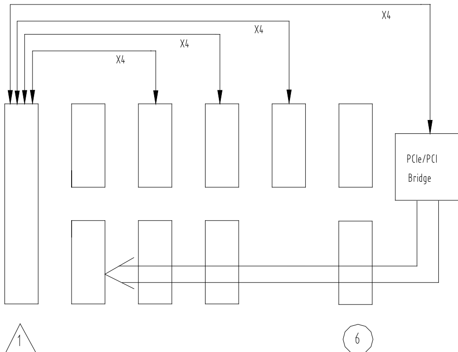
图 4 总线拓扑图
