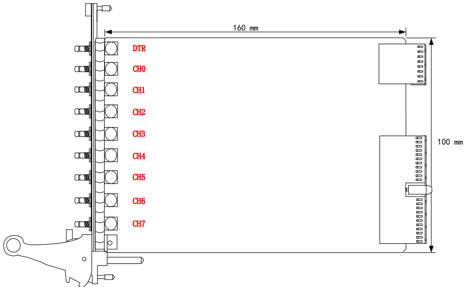
图 3-2-1 PXI8814/8811 板卡尺寸图
