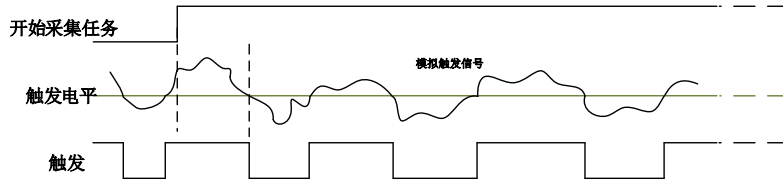
图4-8-6 模拟边沿触发--下降沿触发
