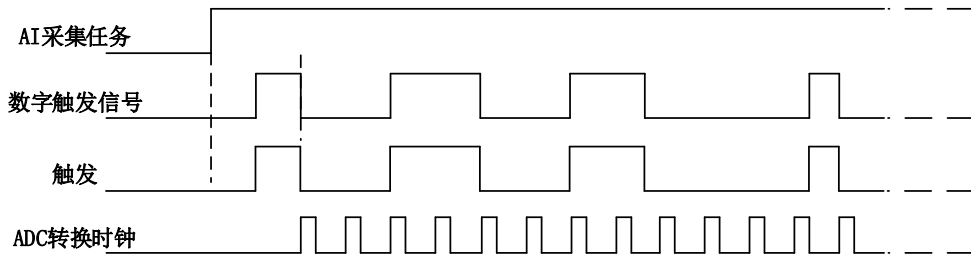
图 4-7-3 数字触发--下降沿触发
