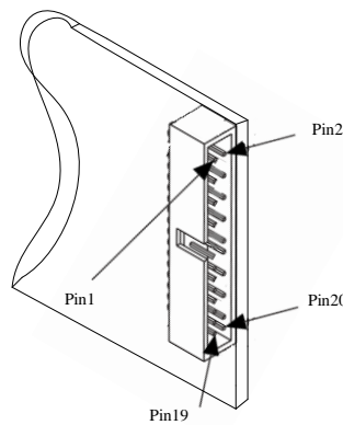
图 3-2-3 RTSI 的 Pinout 图
