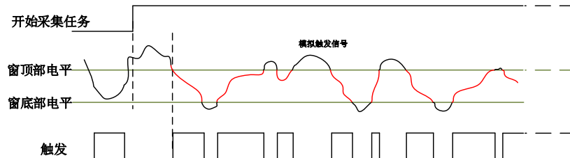
图4-8-8 模拟窗触发--入窗
