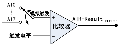
图4-8-5 比较器
