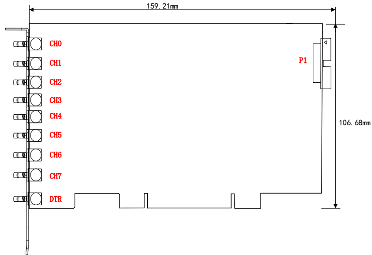
图 3-2-1 PCI8814/8811 板卡尺寸图
