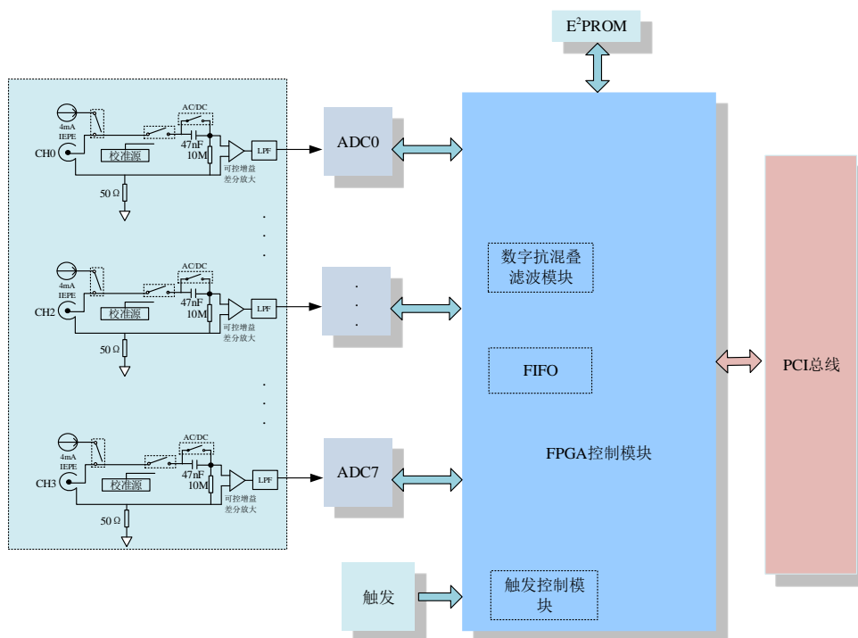
图 2.2.1 PCI/PXI 8811/8814 系统框图
