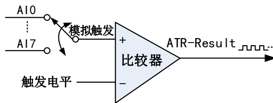
图4-8-7 比较器
