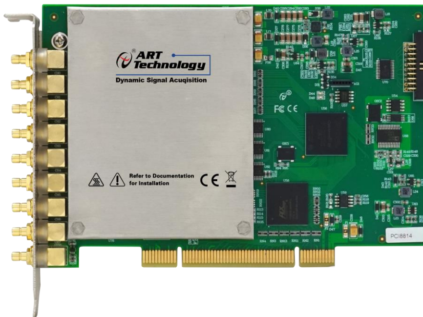
图 3-1-1 PCI8814 外形图
