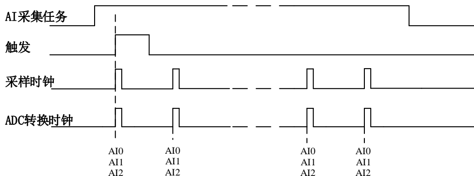
图4-6-3 连续采样
