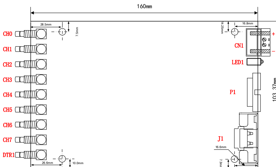
图 3-2-1 板卡尺寸图
