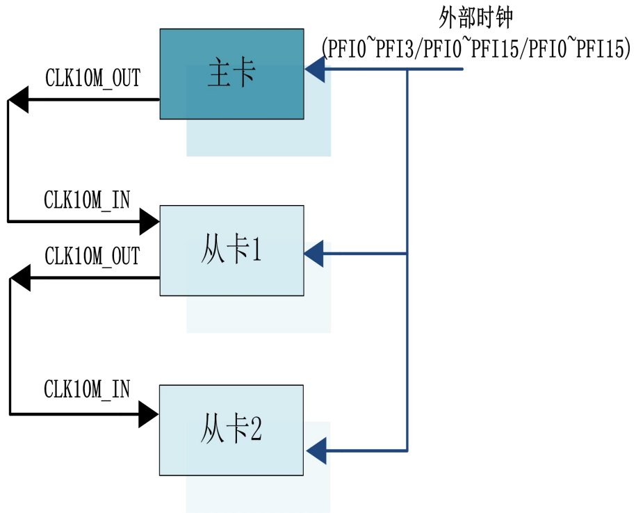
图 4-9-2 共同外时钟
