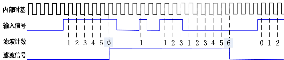
图 5-9-1 脉冲输出
