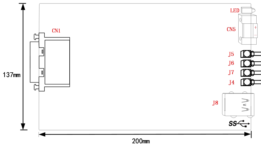
图 3-2-1 板卡尺寸图
