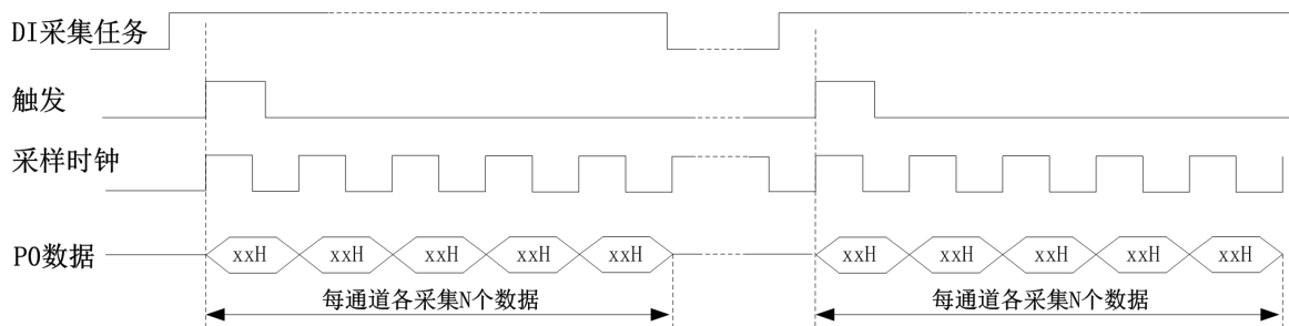
图 6-5-2 有限点采样
