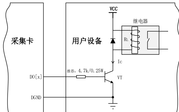
图 7-3-1 DO 数字量控制继电器电路
