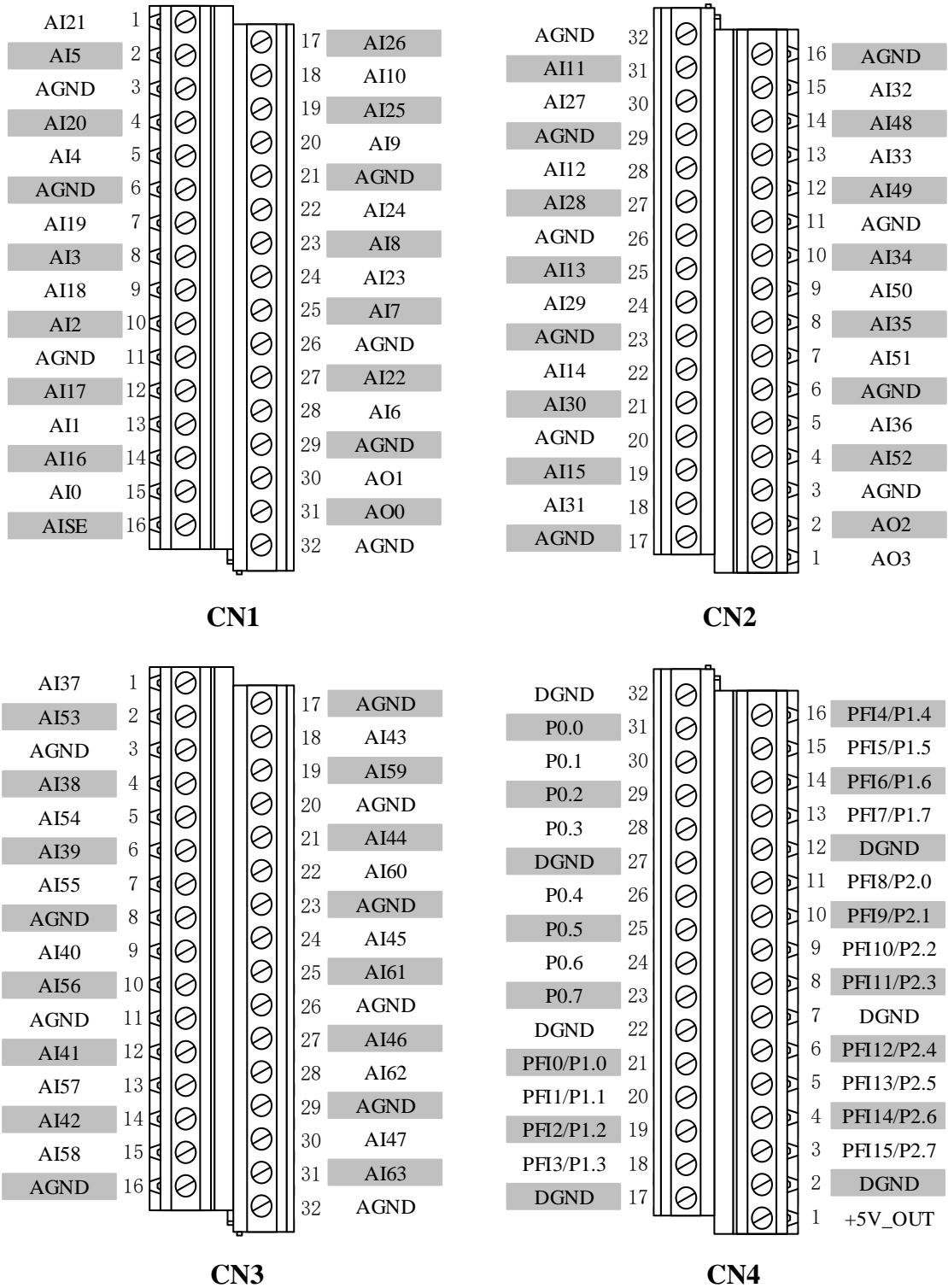
图 3-3-1 USB2861-D 管脚定义
