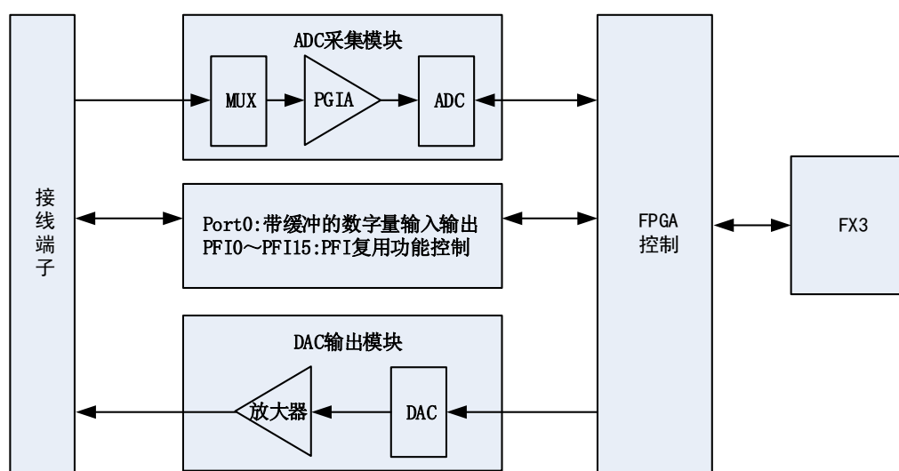
图2-2-1 USB2861系统框图
