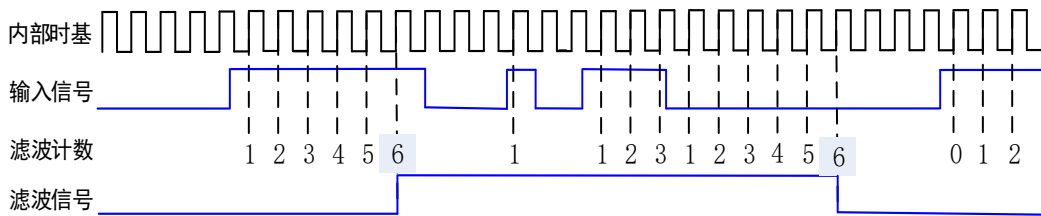
图 6-9-1 脉冲输出
