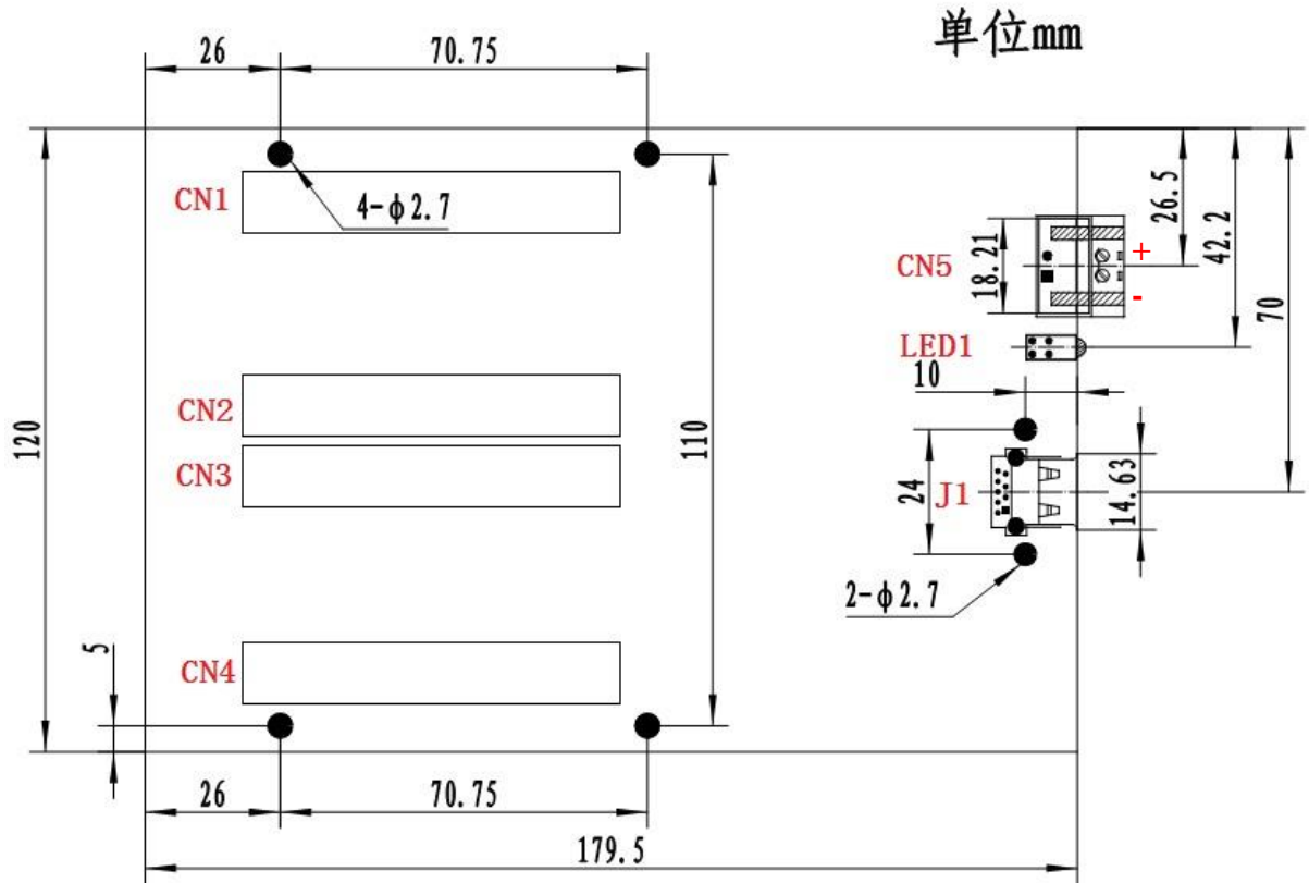
图 3-2-2 板卡尺寸图
