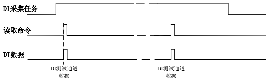
图7-5-1 按需单点采集
