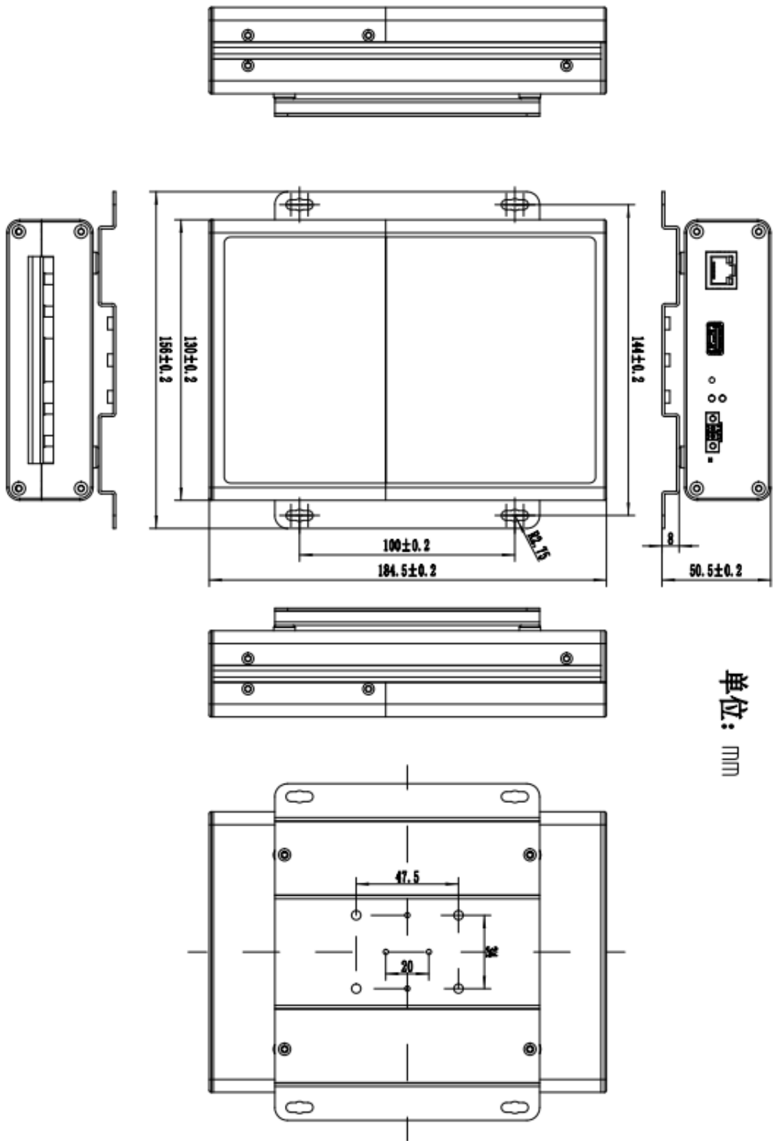
图 3-2-1 外壳尺寸图
