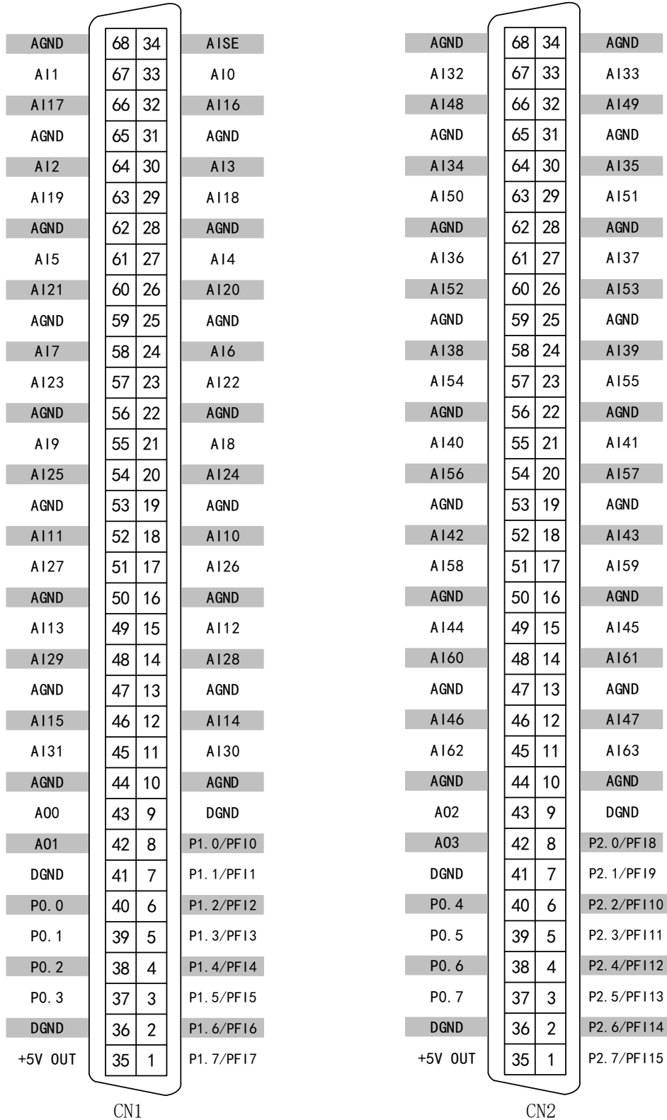
图3-3-2 USB2861-V 管脚定义
