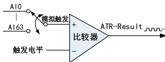
图8-3-4 模拟触发比较器
