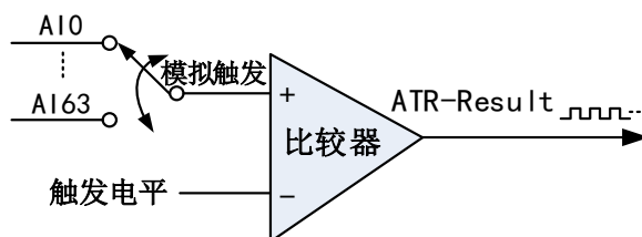
图8-3-6 比较器
