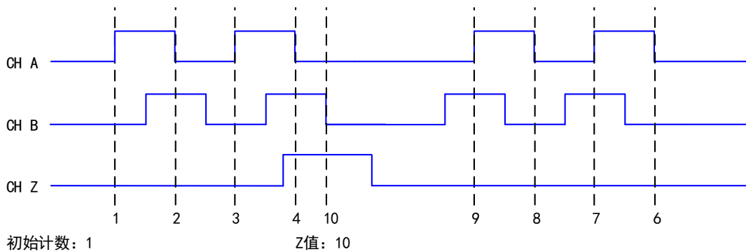
图 6-7-6 Z 索引
