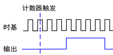
图 6-8-1 单脉冲生成
