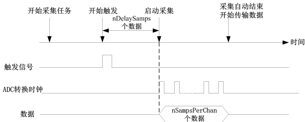
图 4-10-3 硬件延时触发
