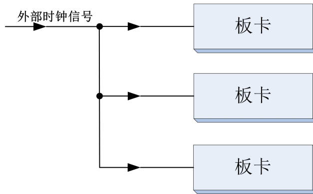
图4-11-3 外时钟同步采集的连接方式
