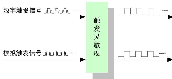
图 4-9-2 触发灵敏度
