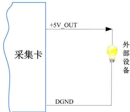
图 8-1-1 +5V 输出接线图
