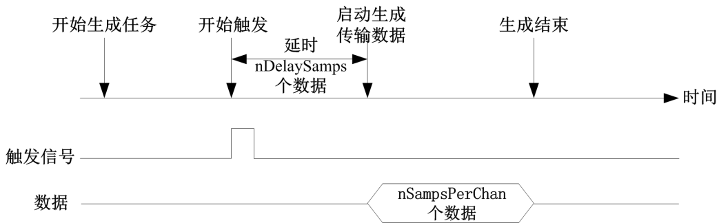
图 5-9-1 延时触发
