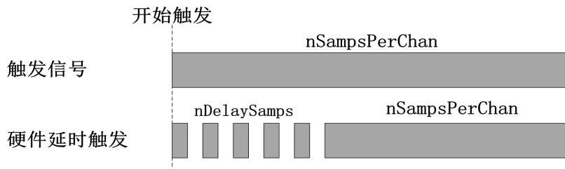
图 4-10-1 AI 触发模式
