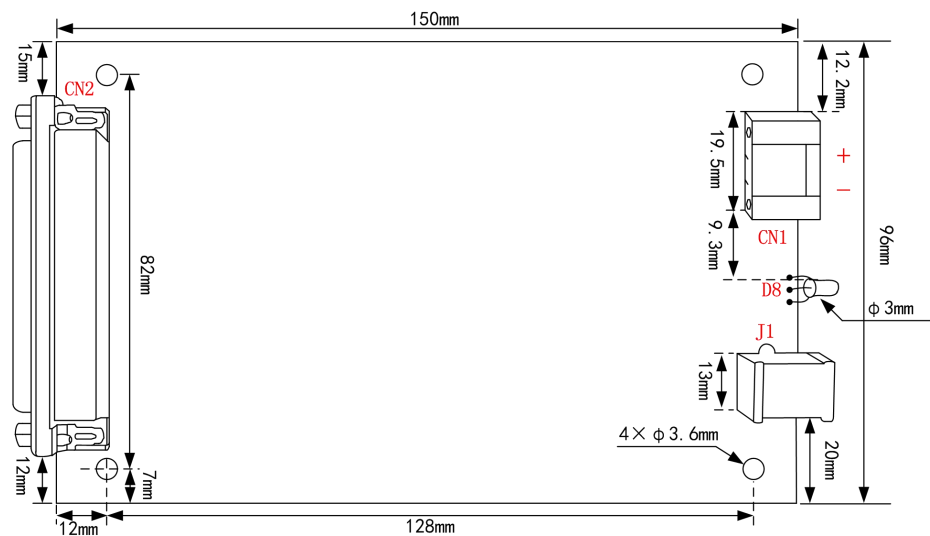
图 3-2-1 板卡尺寸图
