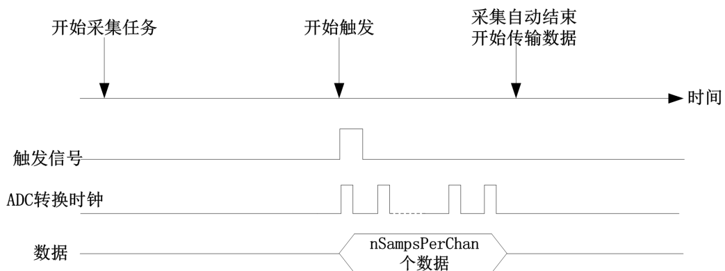
图 4-10-2 开始触发
