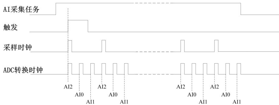
图4-8-4 内时钟连续采样
