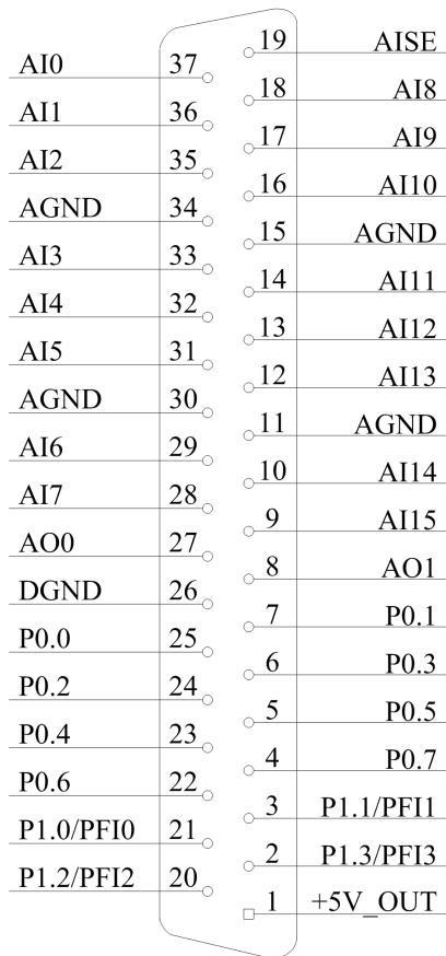
图3-3-1 CN2管脚定义
