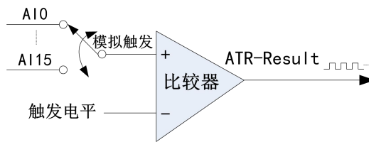
图4-9-5 比较器
