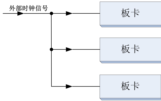
图5-10-3 外时钟同步采集的连接方式
