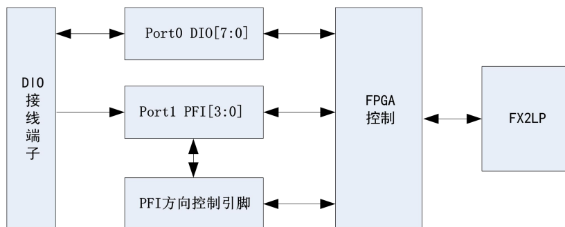
图7-1-1 DIO功能框图
