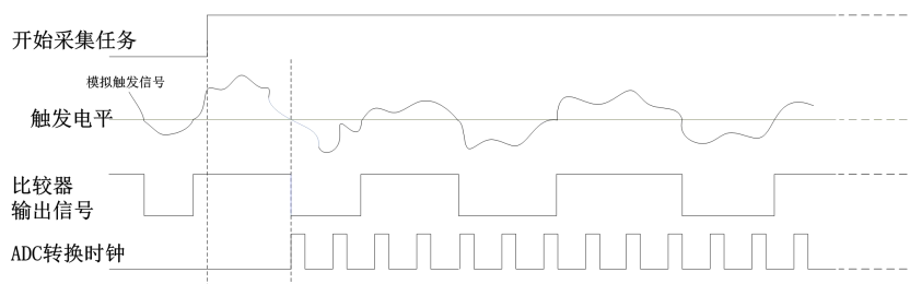
图4-9-6 模拟触发--下降沿触发
