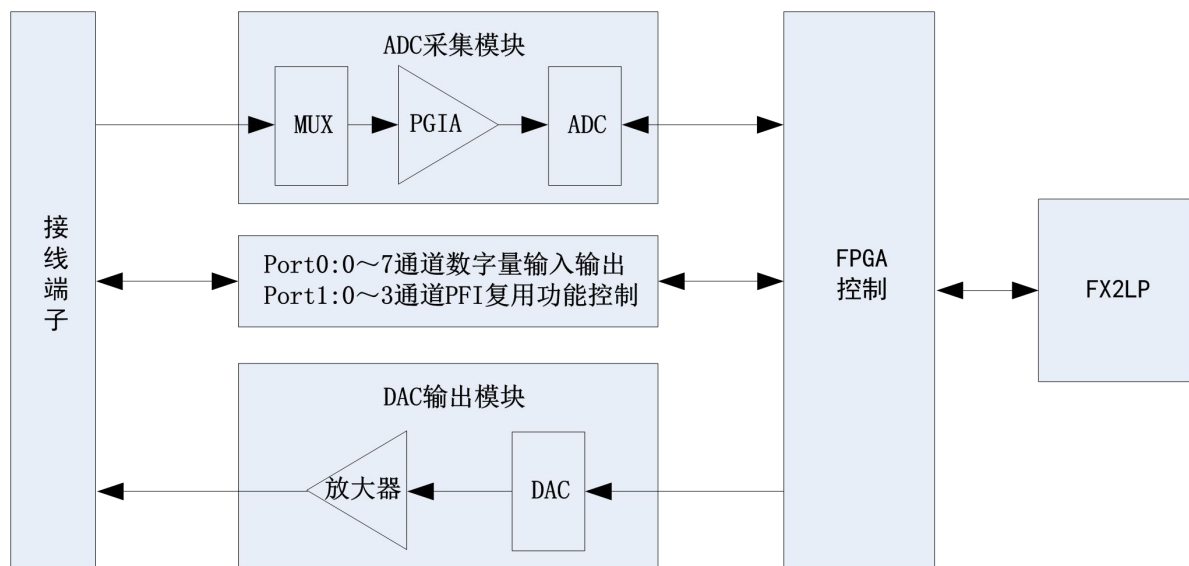
图 2-2-1 USB3101/2/3/6 系统框图
