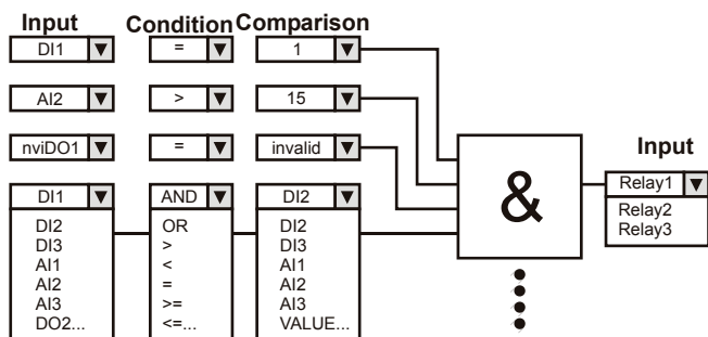
图 1: 开关逻辑功能图
