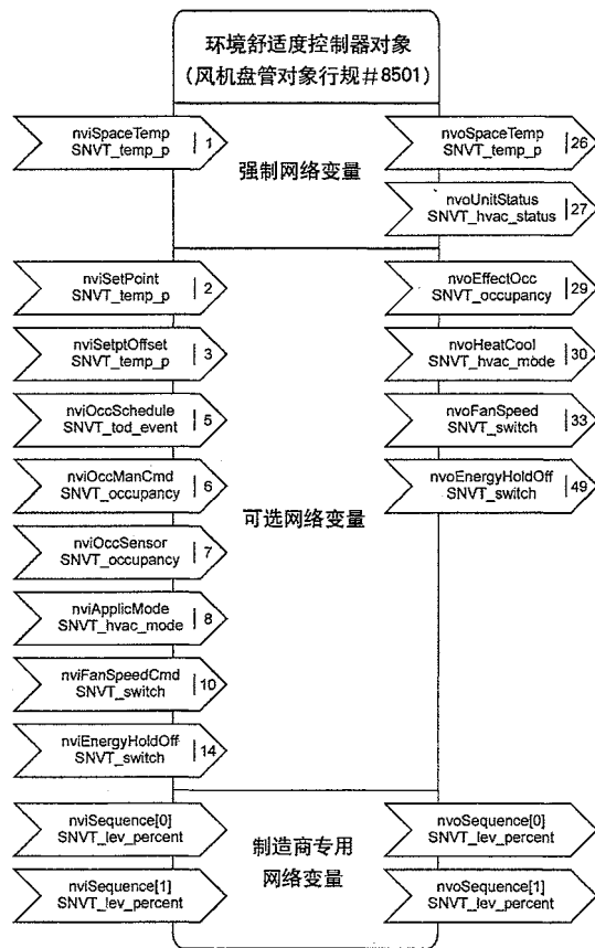
图 4. 环境舒适度控制器对象
