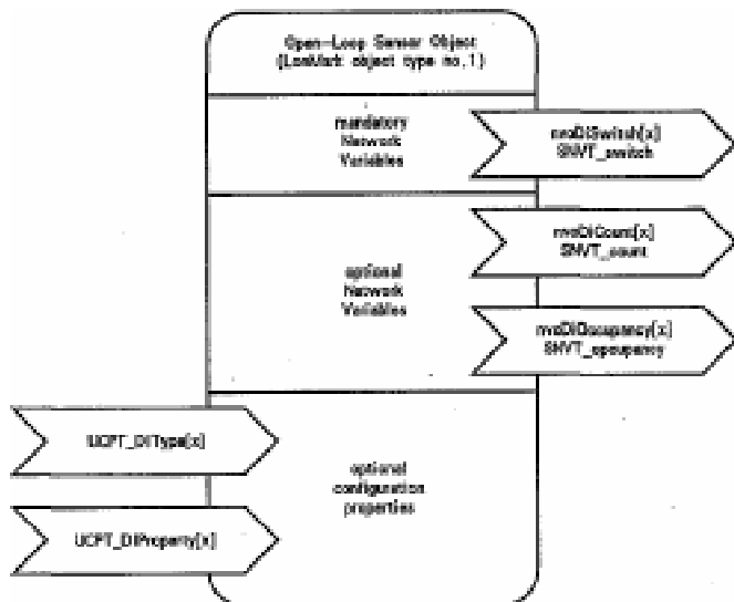
图三. 用于 DI 的 LonMark 传感器对象规范
