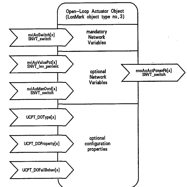
图五. 用于继电器的 LonMark 执行器对象规范
