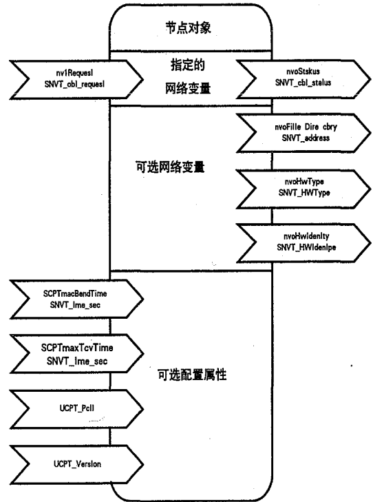
图一. LonMark 节点对象规范
