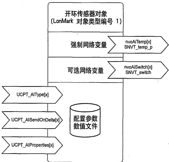
图 7 LONMARK UI 传感器对象行规说明
