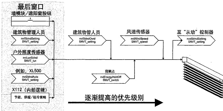
图 9 由 Excel 12 接收 / 读取的遮阳窗输入信号的优先级别
