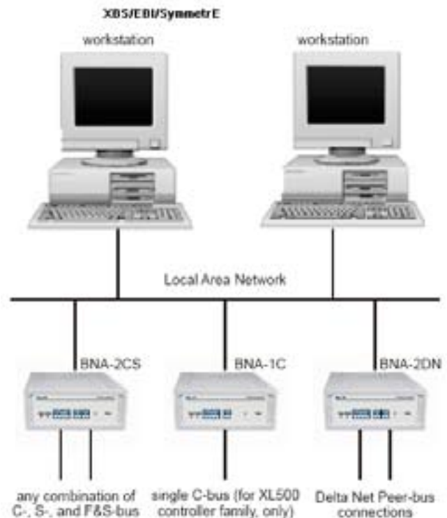
图 1. 应用示例, 结构图
