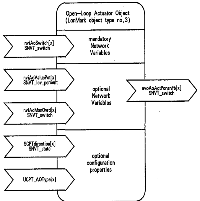
图三. 用于 DI 的 LonMark 传感器对象规范
