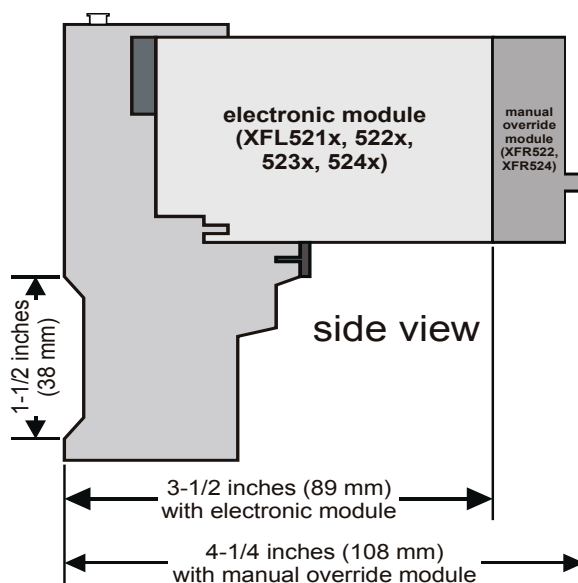
端子块侧视图
