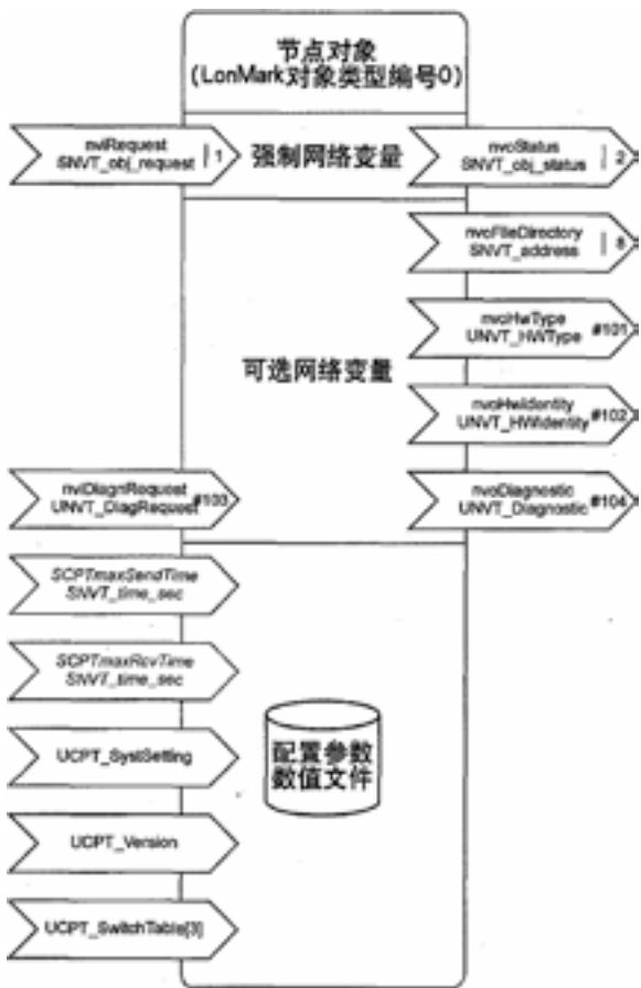
图 6 LONMARK 节点对象规范说明 LONMARK 传感器 / 执行器对象
