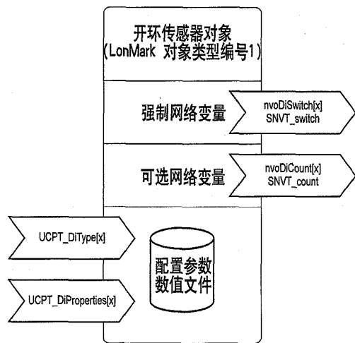
图 8, LONMARK DI 传感器对象行规说明
