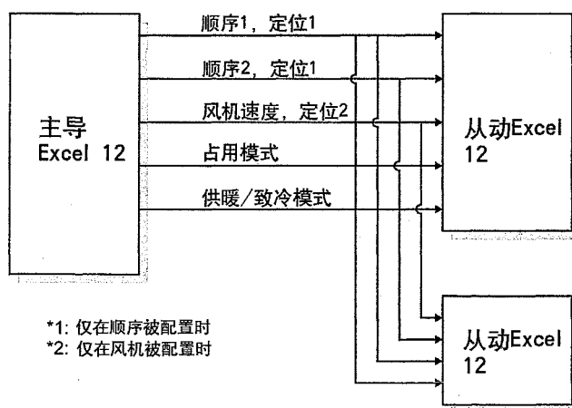
图 2 主 / 从控制功能性:
