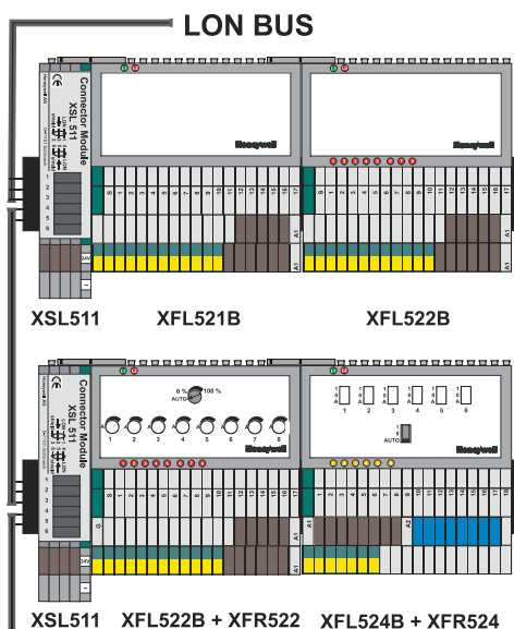
LonWorks连接器端子
