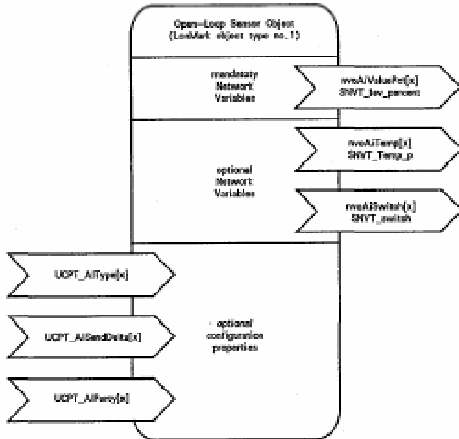
图二. 用于 UI 的 LonMar 传感器对象规范
