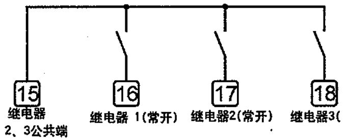
图 4. 继电器输出
