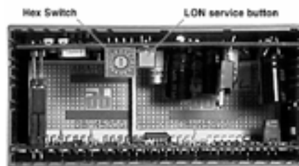
十六进制选择开关(0~F)
