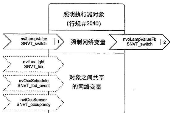
图 5. 照明执行器对象 LONWORKS 网络接口
