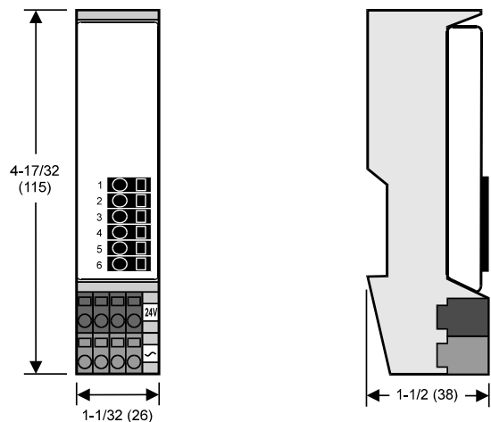
连接器模块XCL511
