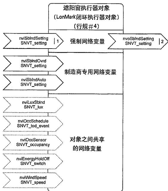
图 7. 遮阳窗执行器对象
