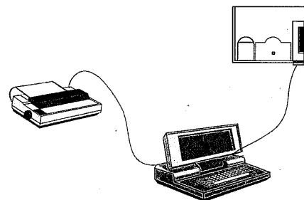
图 2. 配备 XL-ONLINE ( 或 XI584) 和打印机的 Excel500(XCL5010)
