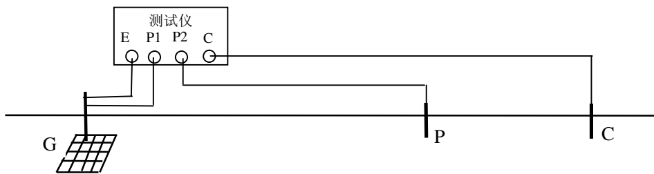
G —被试接地装置 C —电流极 P—电位 图 3 接地阻抗测试接线示意图
