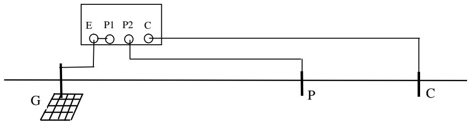
图 2 接地电阻测试接线示意图
