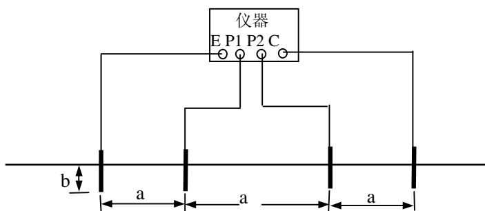
图 5 四极法测量土壤电阻率接线图
