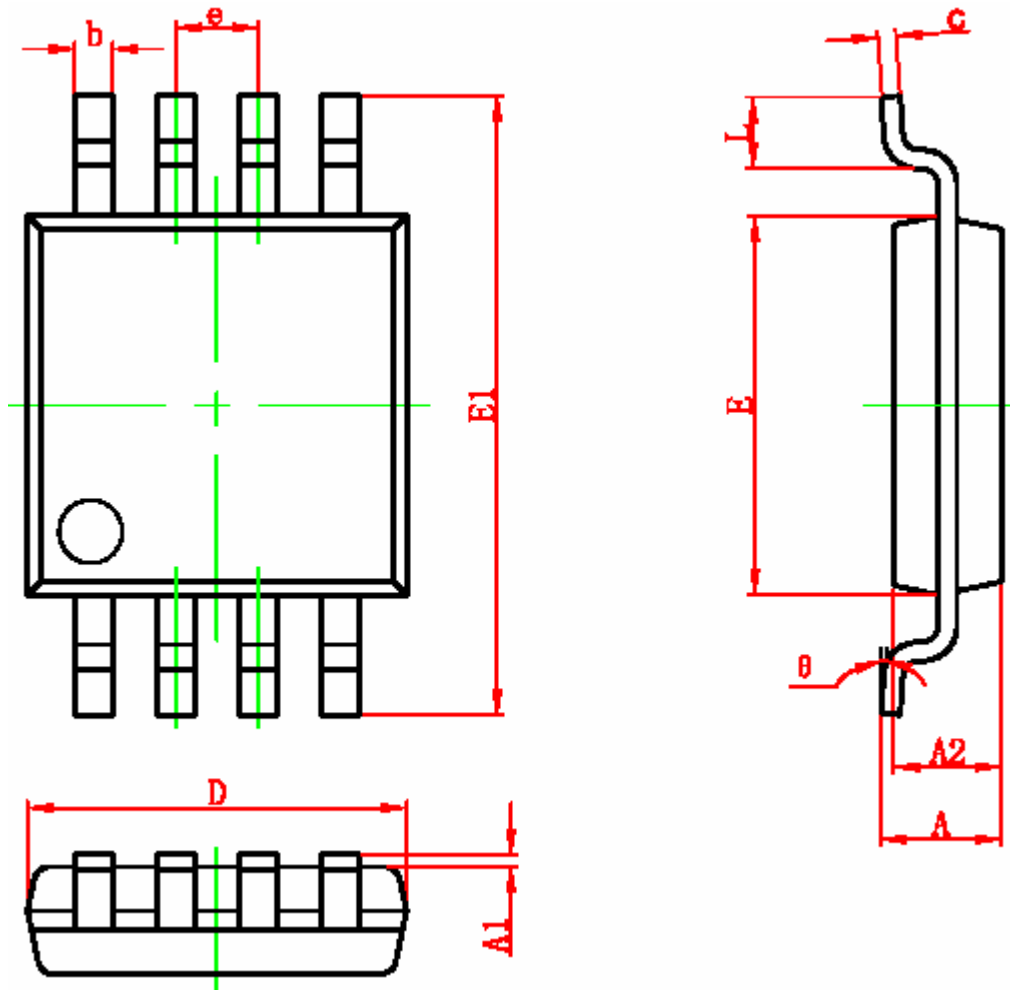
8 引脚 MSOP-PP 封装 (单位 mm)
