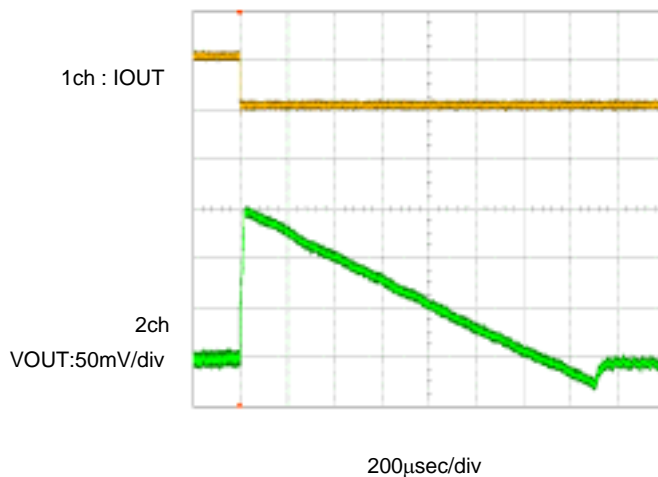
IOUT=300mA ⇒ 0.1mA
