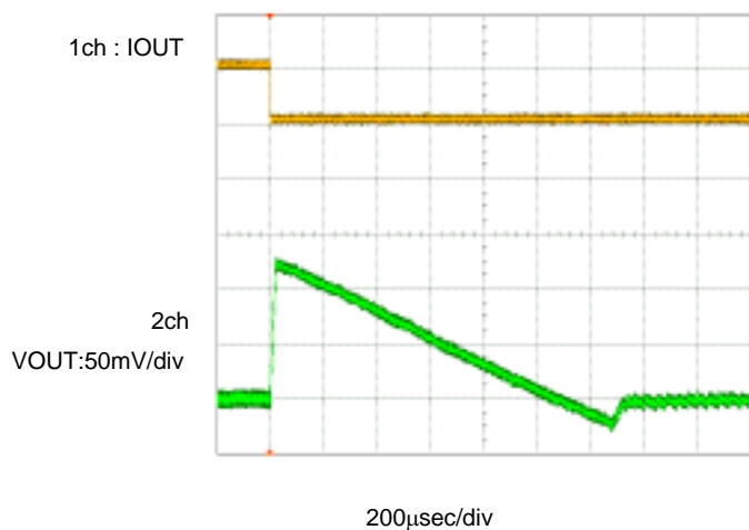
IOUT=100mA ⇒ 0.1mA
