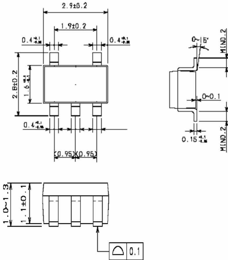
SOT-23-5L
