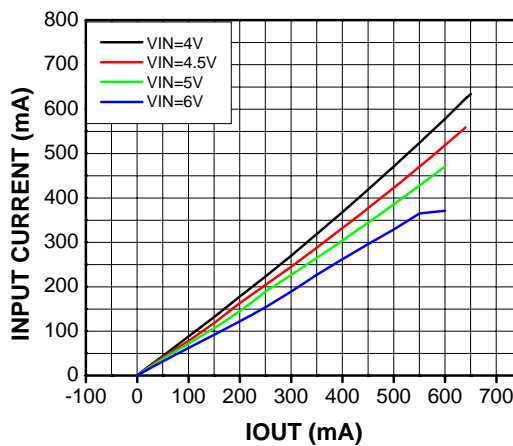
(3) 输入电流随输出电流的变化
