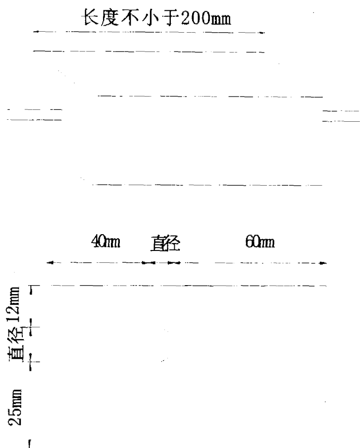
图 A.0.1 校准试件示意图
