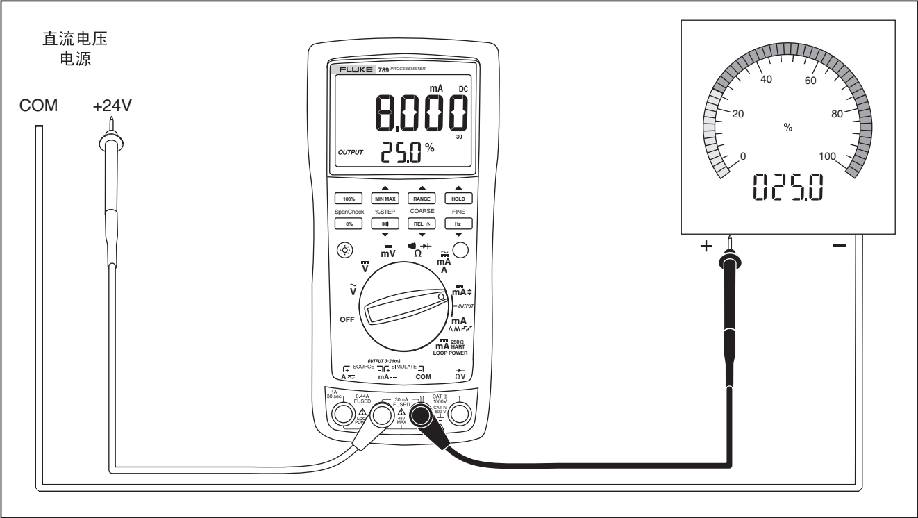
图 8。模拟变送器
