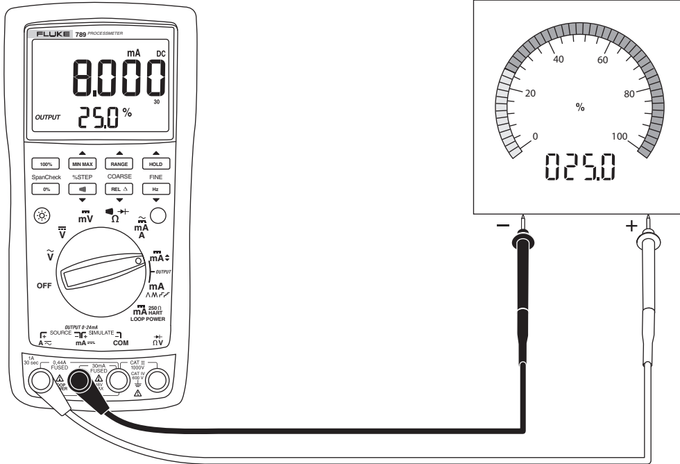
图 7. 源电流
