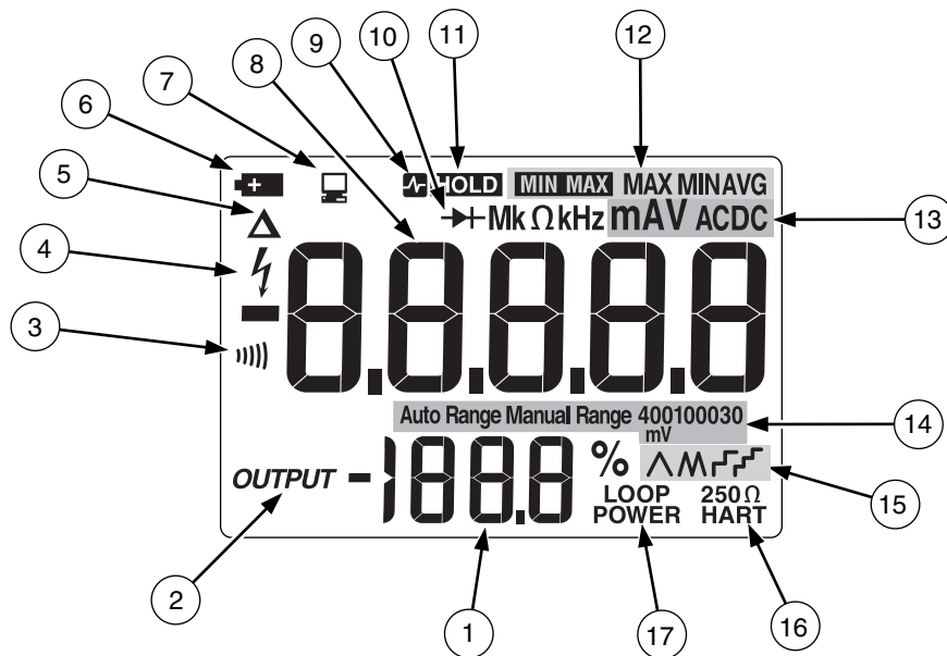
图 6。显示单元
