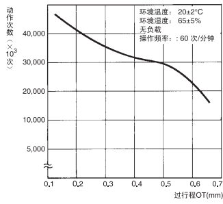
机械寿命曲线 (针状按钮型) SSG-5型
