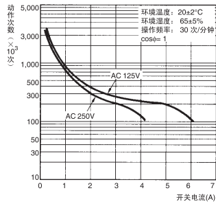
电气寿命曲线 (针状按钮型) SSG-5型
