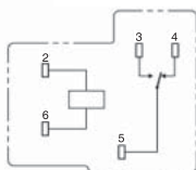
端子排列/外部接口 (BOTTOM VIEW)
