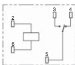
端子排列/外部接口 (BOTTOM VIEW)
