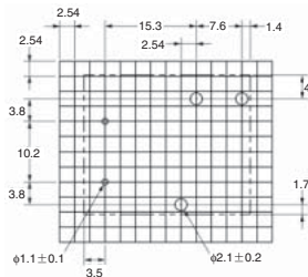
安装孔加工尺寸 (BOTTOM VIEW)
