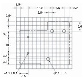
安装孔加工尺寸 (BOTTOM VIEW)
