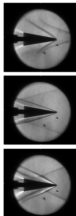
六马赫高超声速静风洞中气流和激波观测
