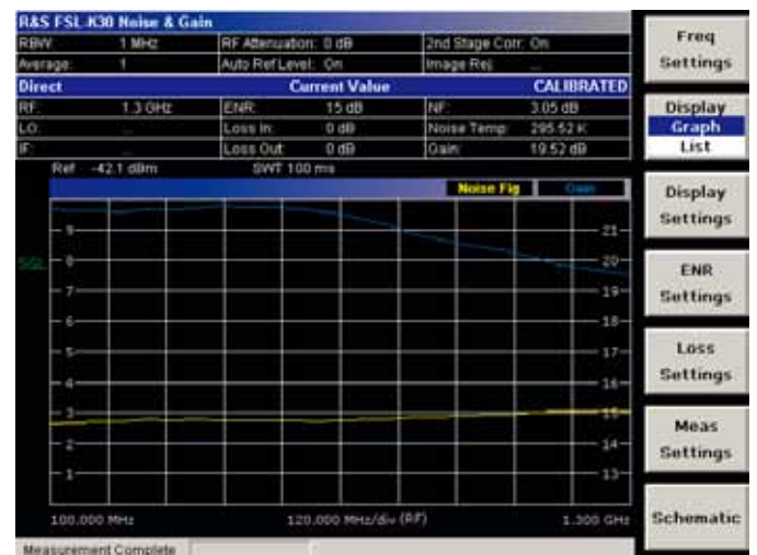
放大器测量
