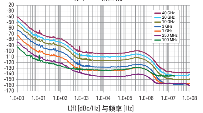
标准 SSB 相位噪声
