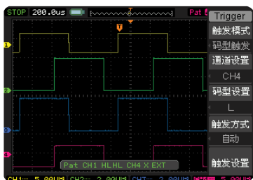
码型触发
