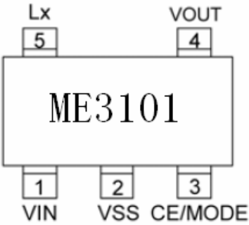
SOT-23-5L
