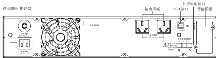
Rack1K 后盖板
