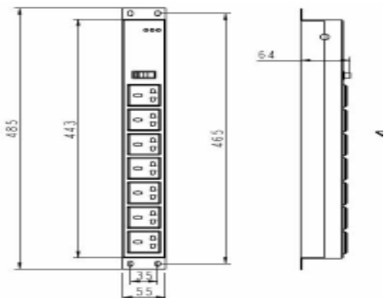
DXH06-Z20/7K 外形尺寸图
