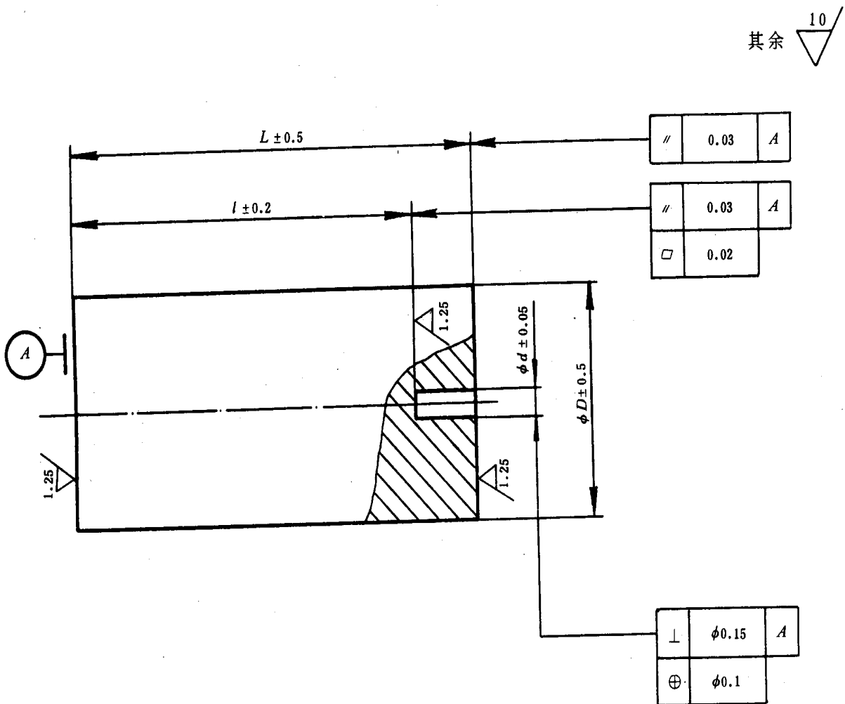
ZGZ 系列对比试块
