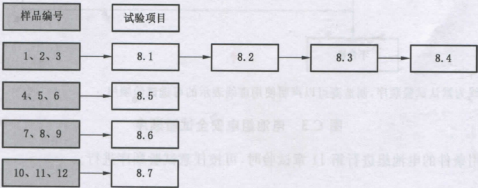
图 C.2 电池组环境安全试验顺序
