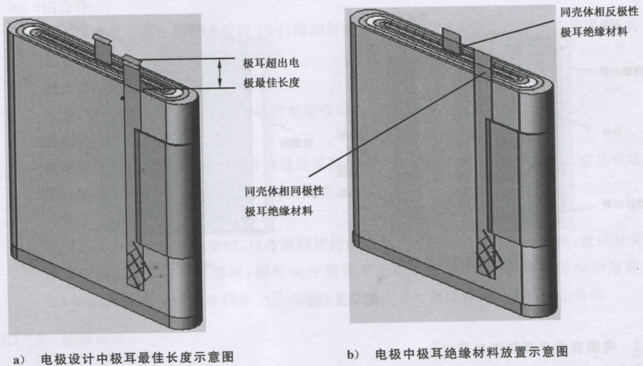
图 B.3 电极中极耳布局
