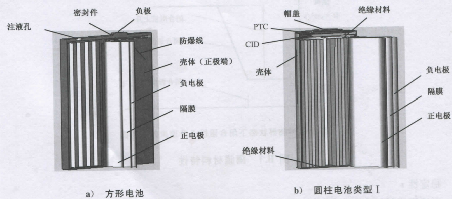
图 B.2 锂离子电池结构实例
