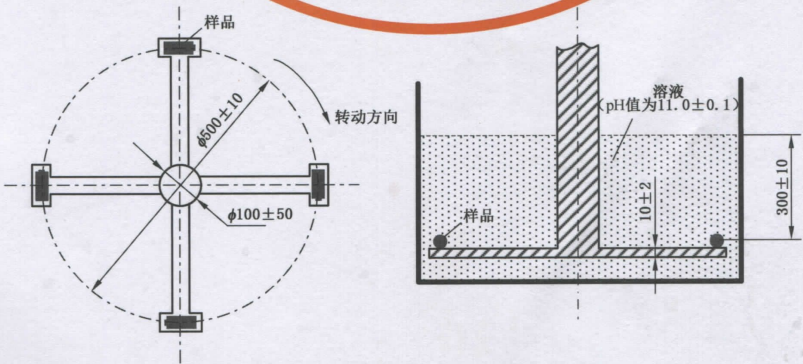
图 E.3 洗涤试验装置
