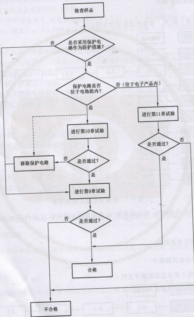
图 C.3 电池组电安全试验顺序
