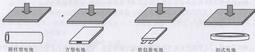
图2 挤压实验中电池放置示意图
