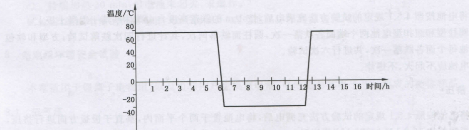
图 1 温度循环流程示意图
