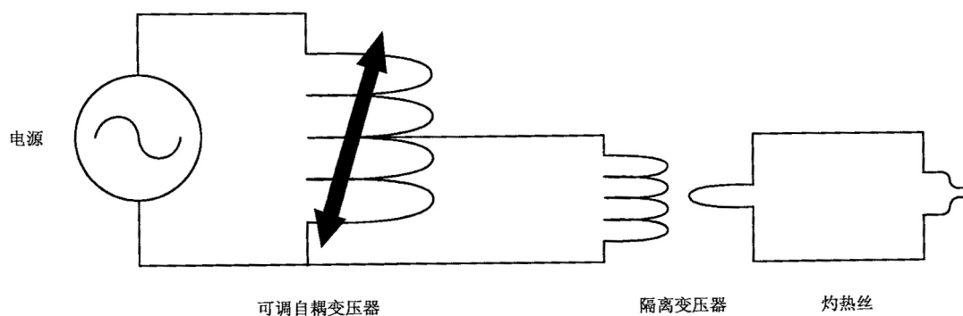
图 2 试验电路
