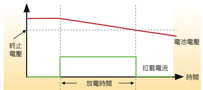
圖 3 電時放電測試
