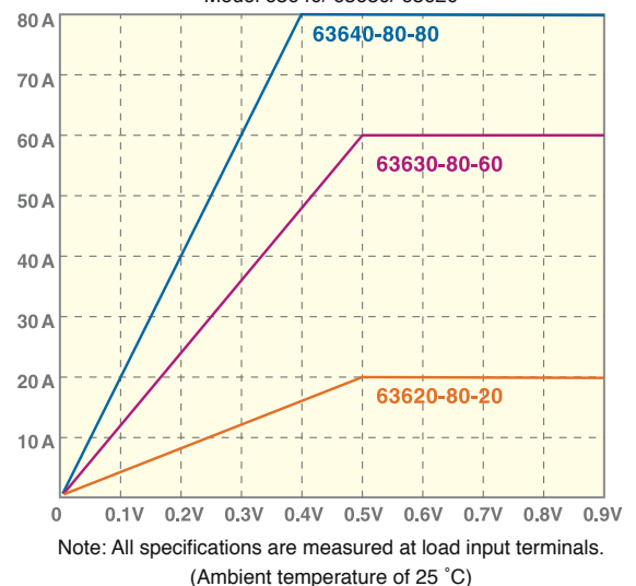
63600系列低電壓 & V-I 曲線操作特性 (Typical) : Model 63640/ 63630/ 63620
