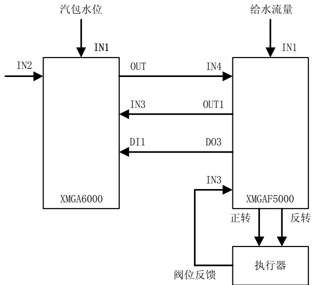
范例1： 锅炉水位三冲量控制接线图
