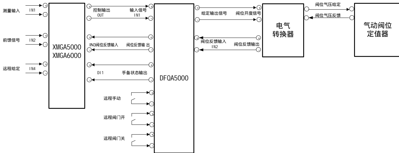
XMGA5000/6000 调节器、后备操作器、电气转换器、气动阀门执行器接线图
