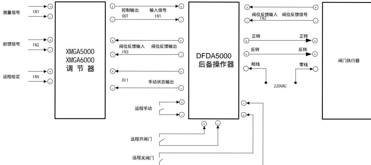
XMGA5000/6000 调节器，后备操作器和电动阀门执行器接线图
