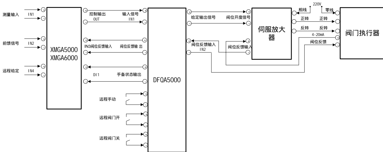
XMGA5000/6000 调节器、后备操作器、伺服放大器、电动阀门执行器接线图
