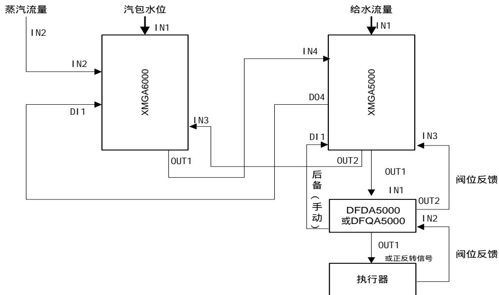
范例1： 锅炉水位三冲量控制接线图
