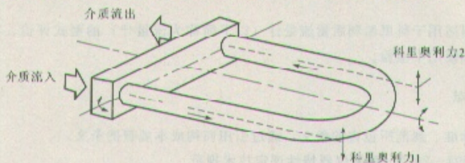
图1 U型振动管的工作原理图
