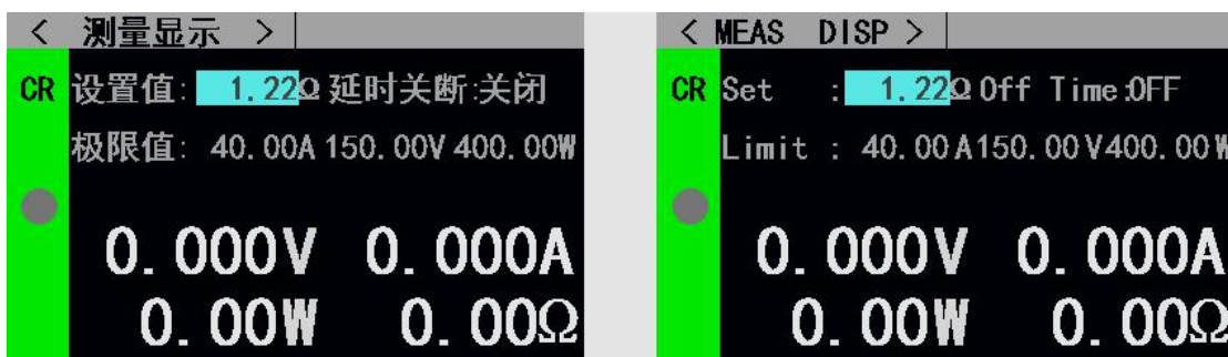
图 2.4.3 定电阻测量模式
