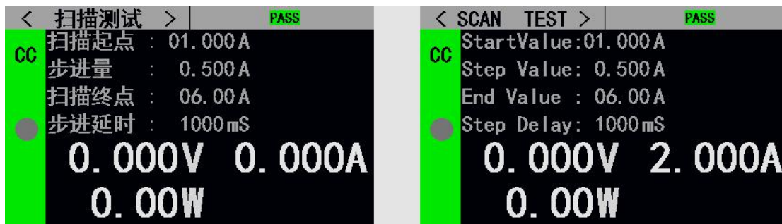
图 2.7.2 扫描测试界面
