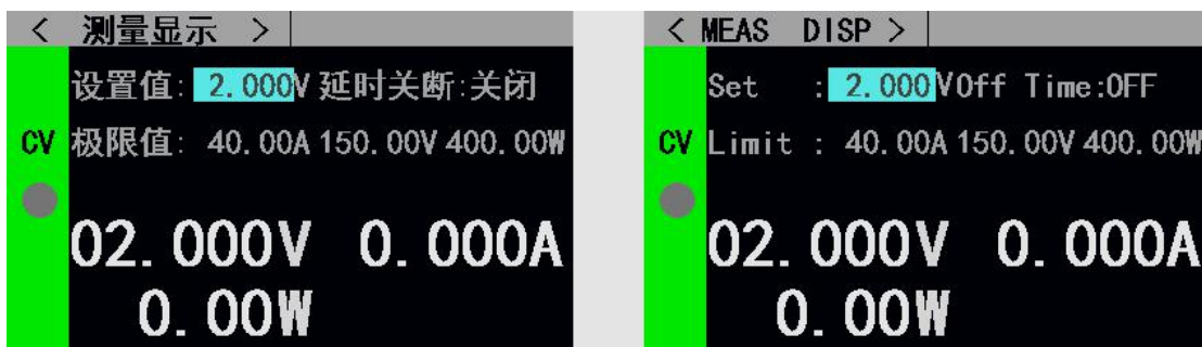
图 2.4.2 定电压测量模式
