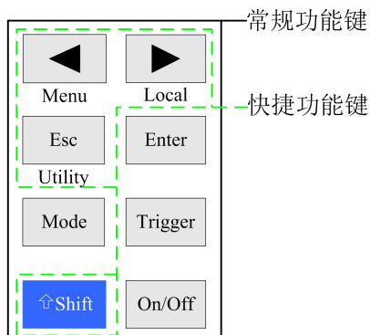
ET5410、5411单通道直流电子负载按键
