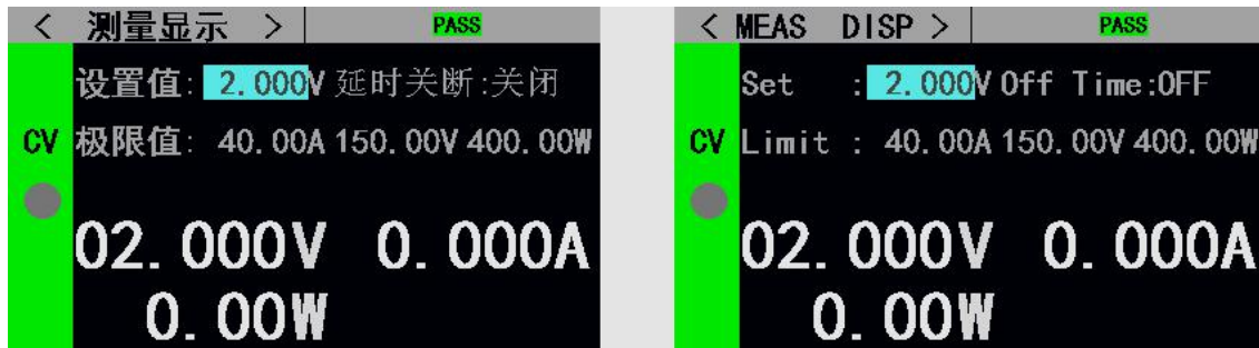
图 2.14.2 开启合格测试后的界面
