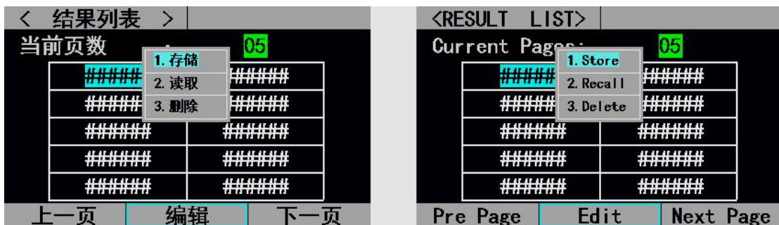
图 2.6.5 文件列表结果保存界面
