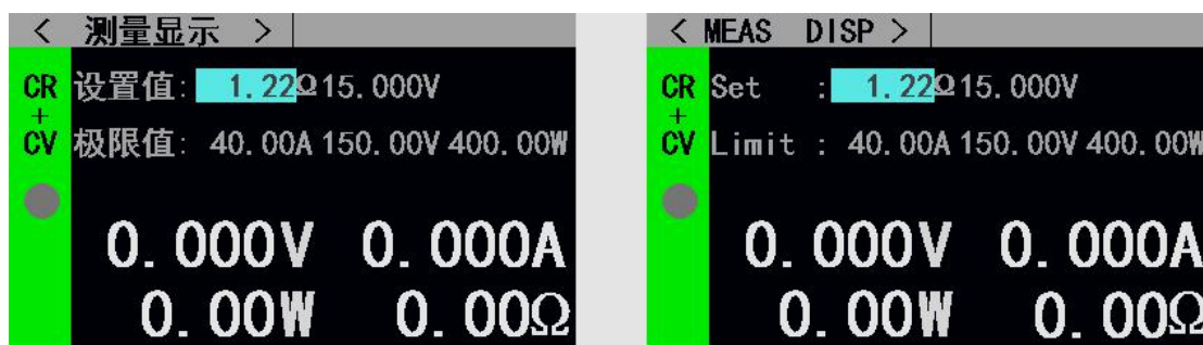
图 2.4.5 定电阻转定电压测量模式
