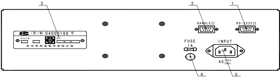
图 1-1 仪器后面板示意图
