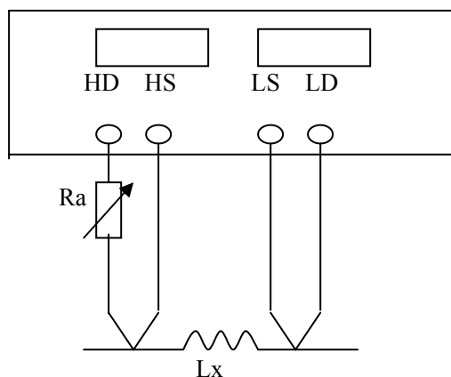
图 3-4 信号源内阻调节示意图
