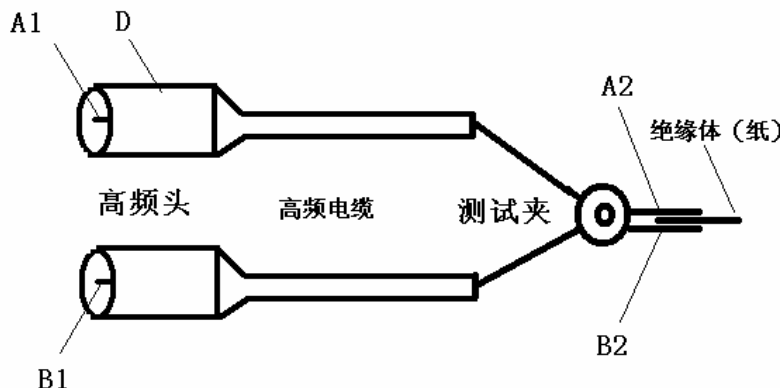
图 3-5 测试电缆局部连线图
