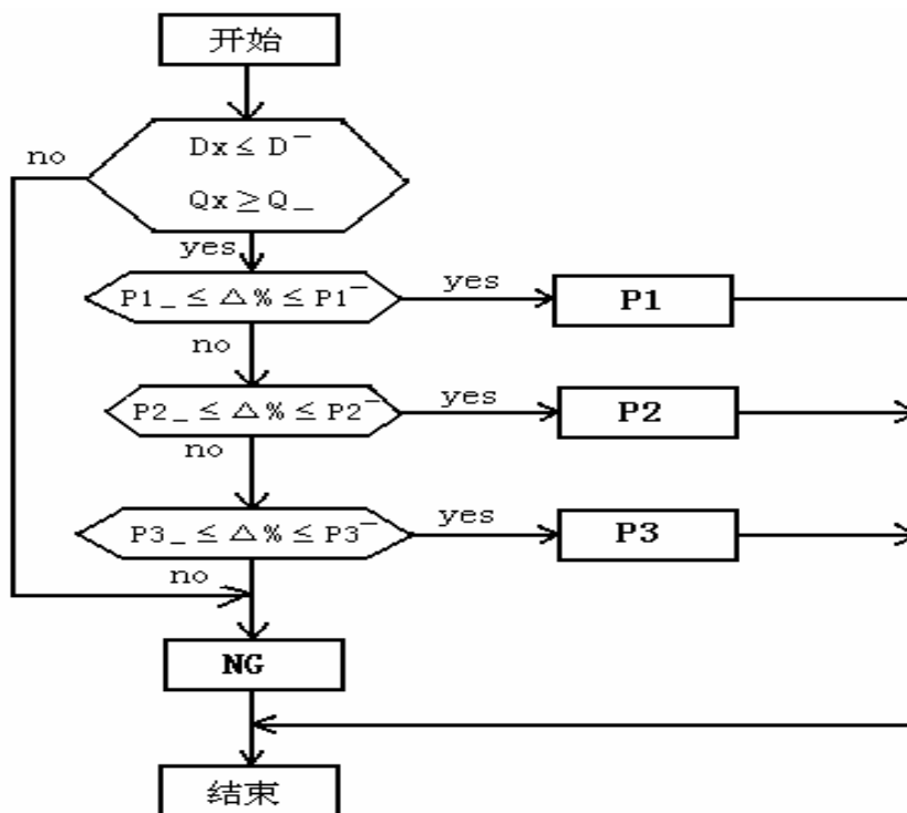
图 2-7 P3 状态的分选判别流程
