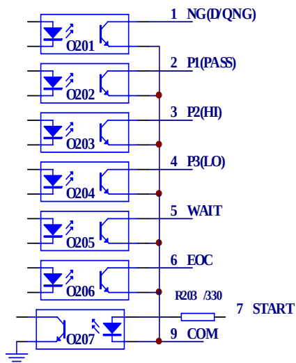
图 2-9 HANDLER 接口引脚图
