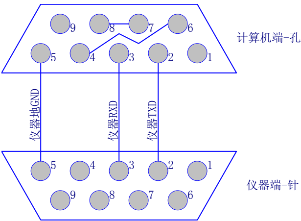
串行通讯电缆连线图
