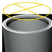
塔架法兰内倾度
