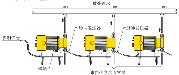
脉冲发送器应用图例
