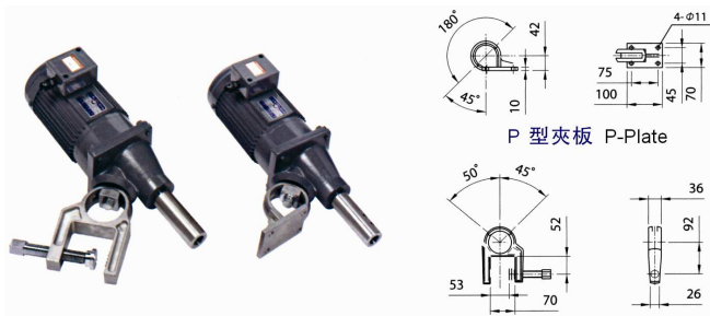
C-018 尺寸表 C-18 Dimension Table
