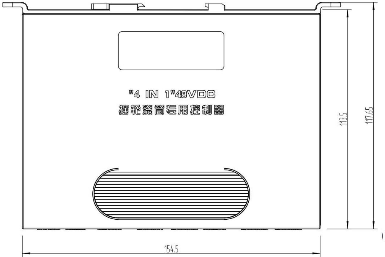
图 2-3 尺寸 2(单位 mm)
