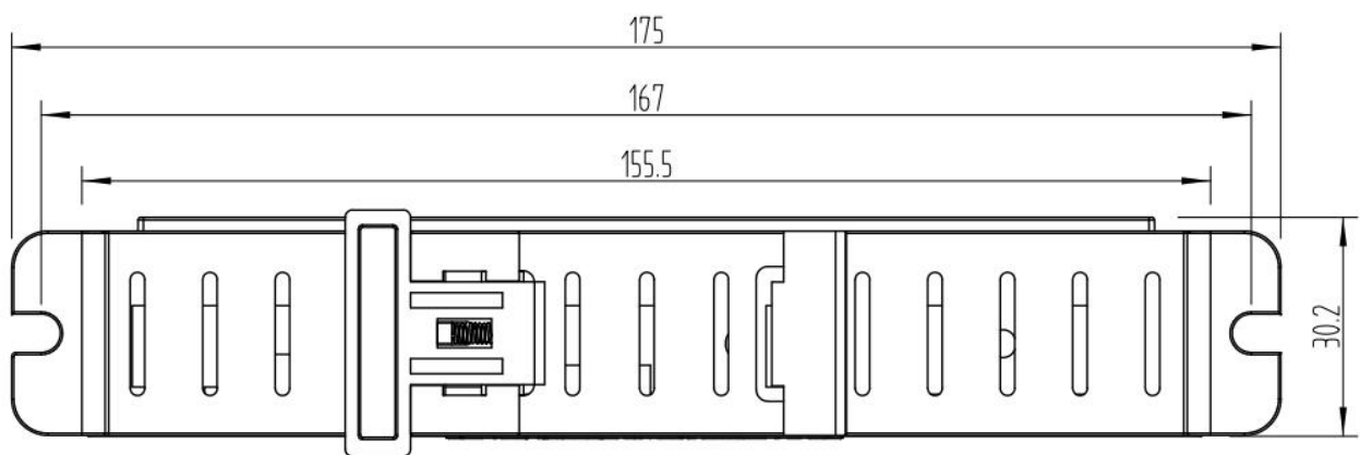
图 2-2 尺寸 1(单位 mm)
