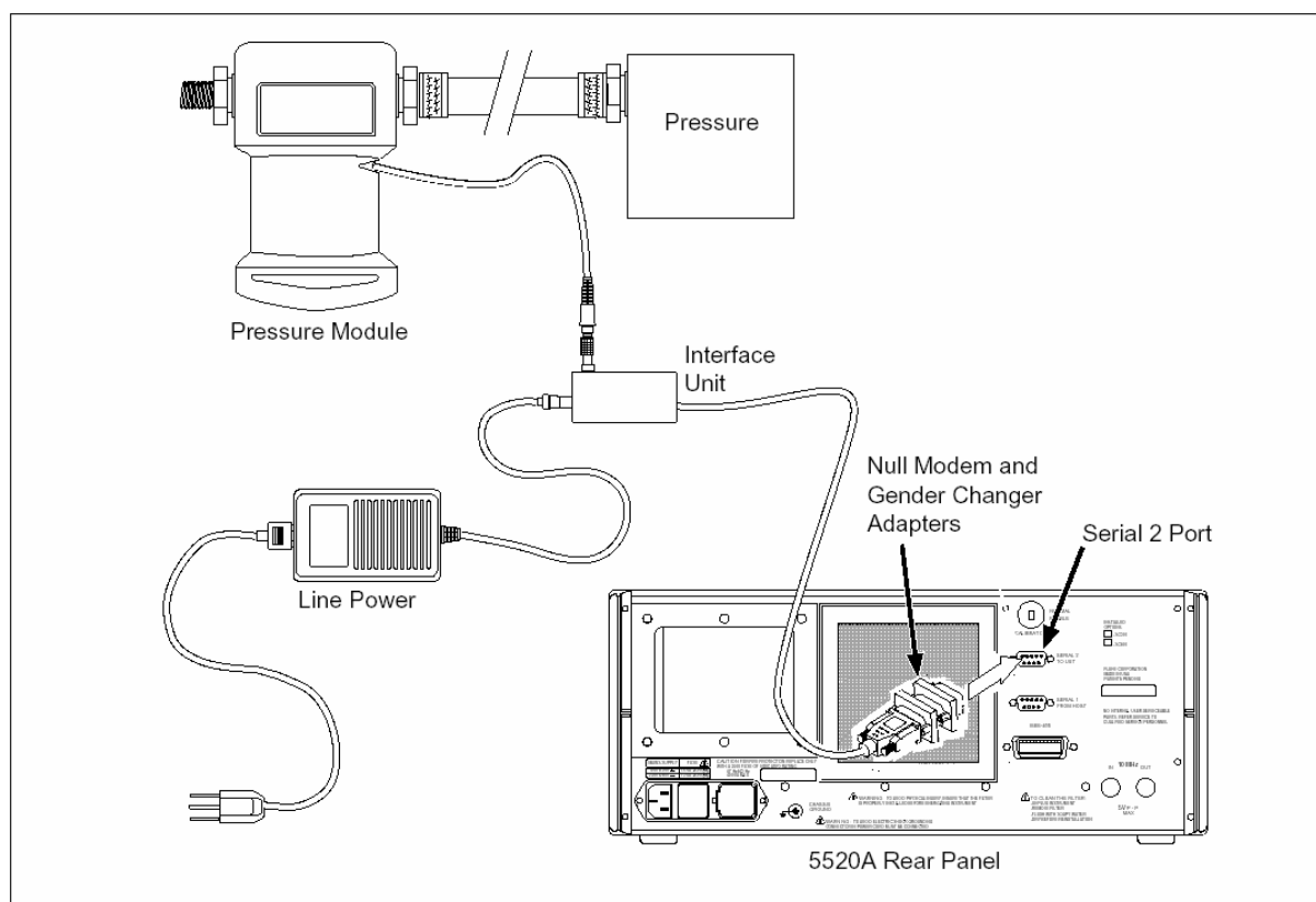
[图 4-15，测量压力]
