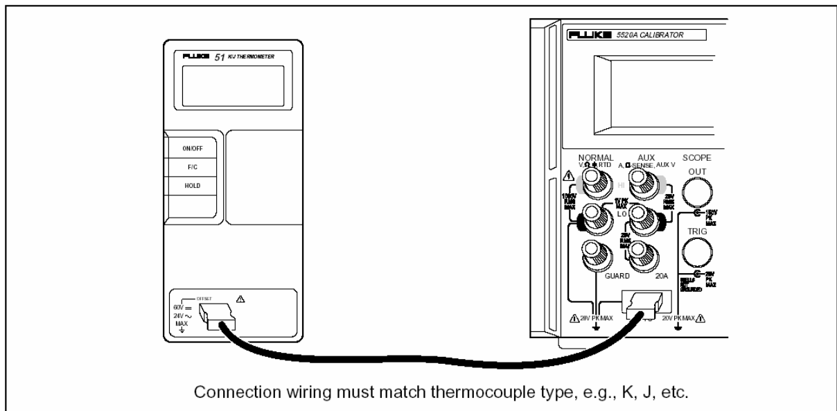
[图 4-10, UUT 的连接: 温度 (热电偶) ]
