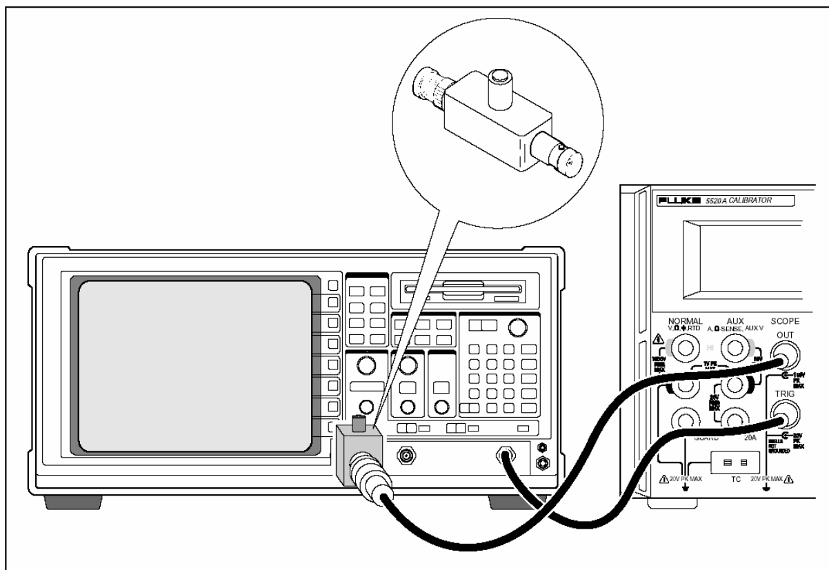
[图 8-2 隧道二极管脉冲器]
