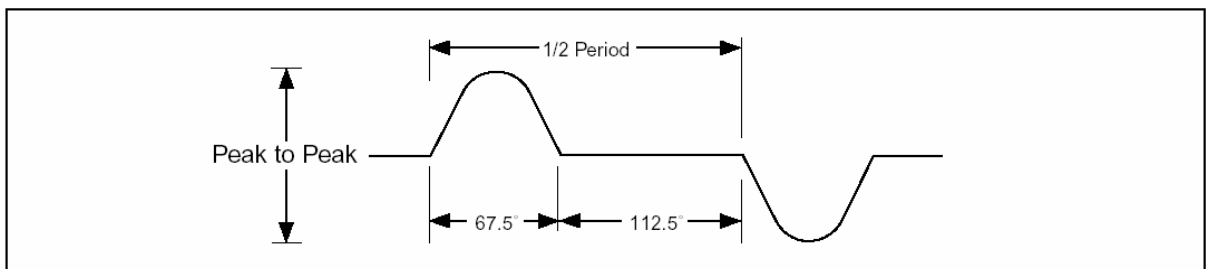
(图 4-14, 截断正弦波)
