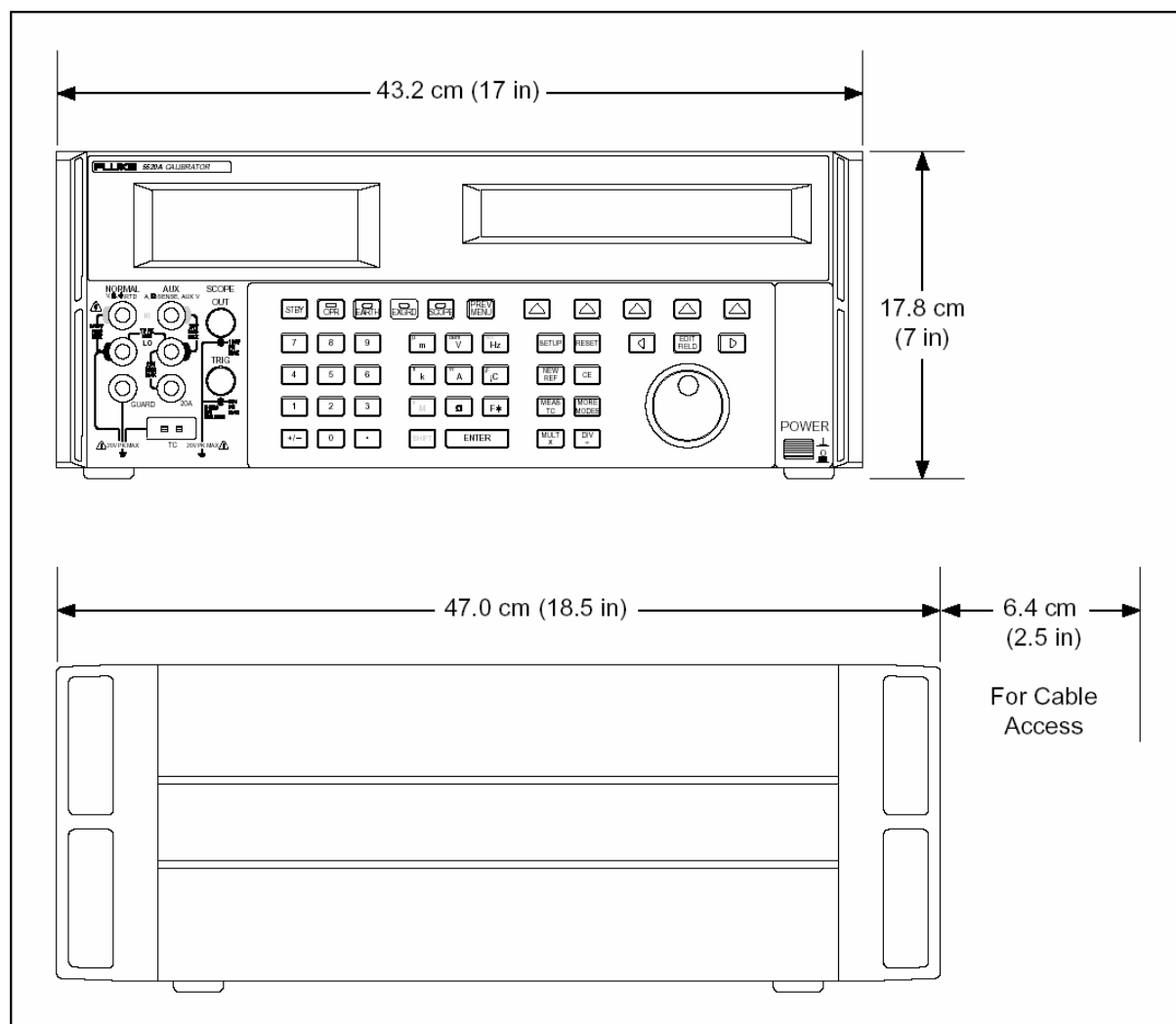
[图 1-3， 5520A 型多产品校准器的外形尺寸]
