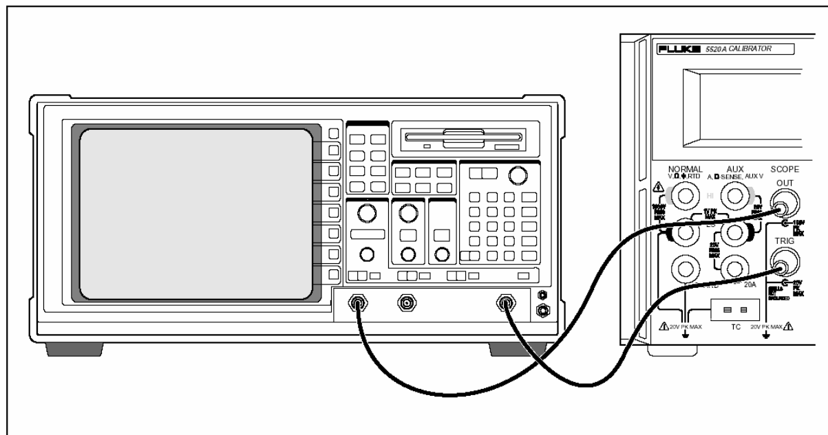
图 8-1 示波器的连接：通道和外部触发
