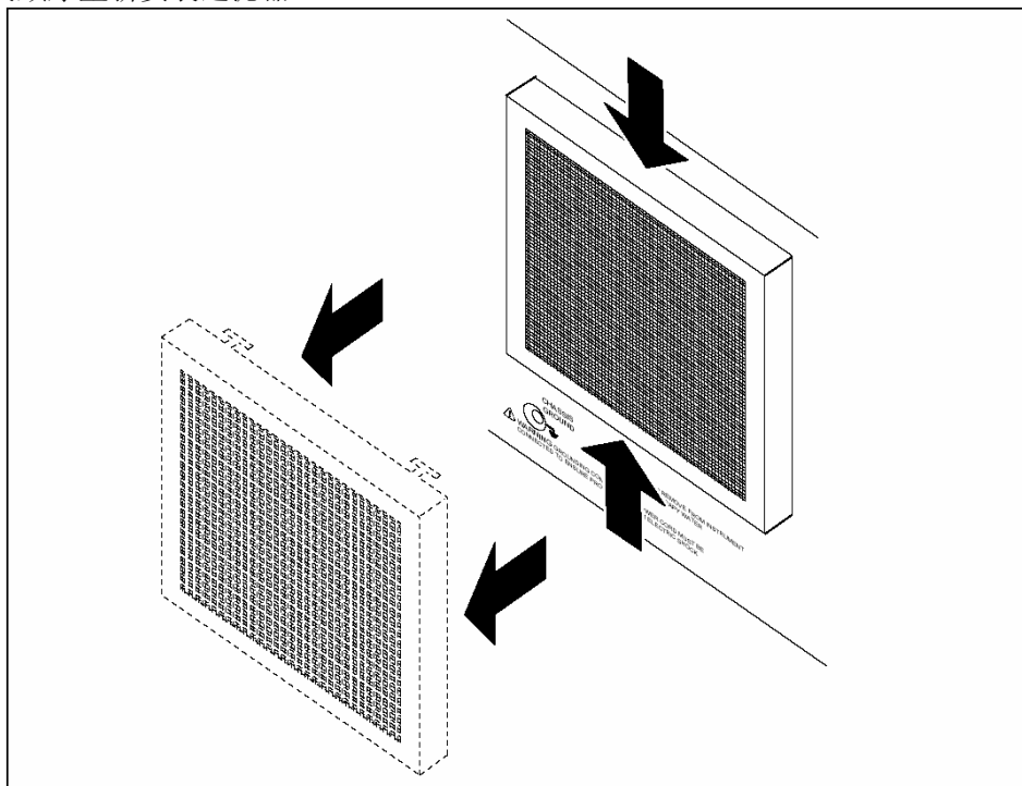
(图 7-2，拆装空气过滤器)
