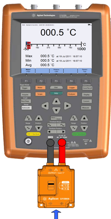
K型热电偶探头
