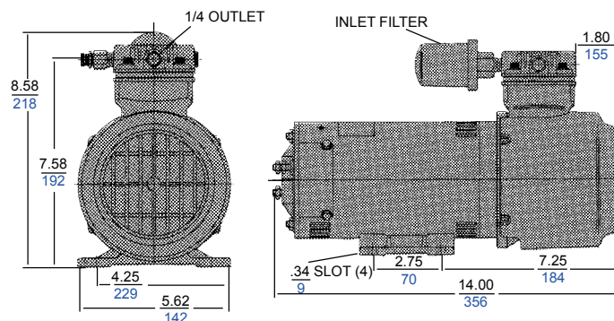
直流单泵头
