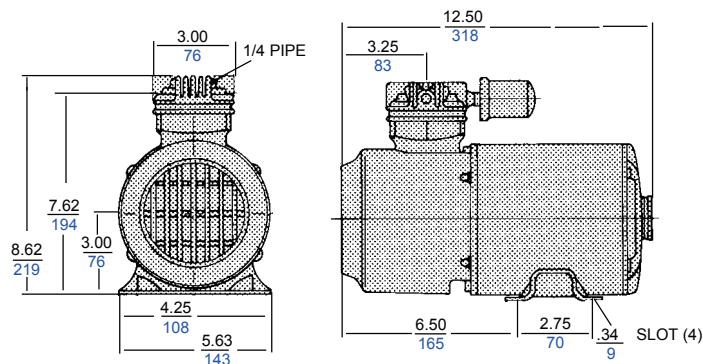
交流单泵头
