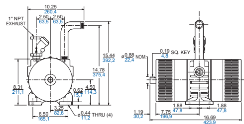
压缩机
