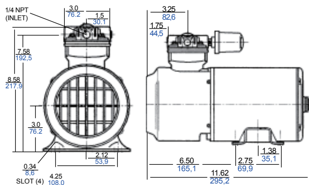
交流电机
