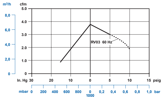
真空泵
