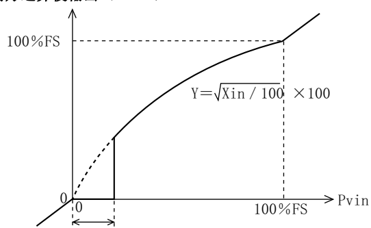
開方運算後輸出 (Pvout)
