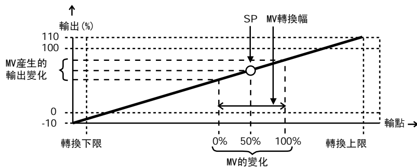
輸出種類為SP+MVの場合
