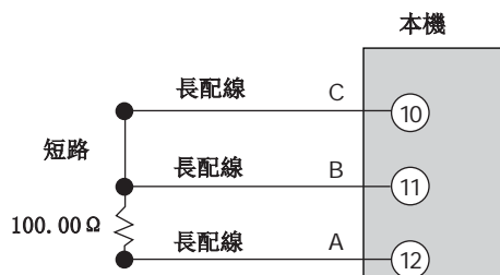
接線狀態 3
