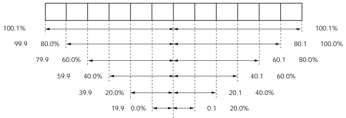
偏差標志的燈亮範圍 (對MS顯示燈偏差範圍的偏差 =PV-SP的比例)
