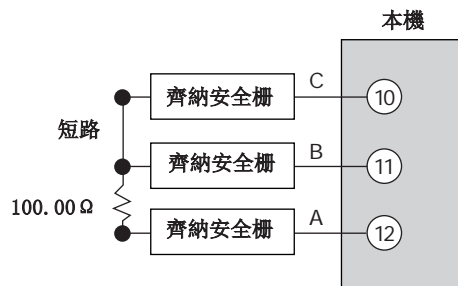
接線狀態 2
