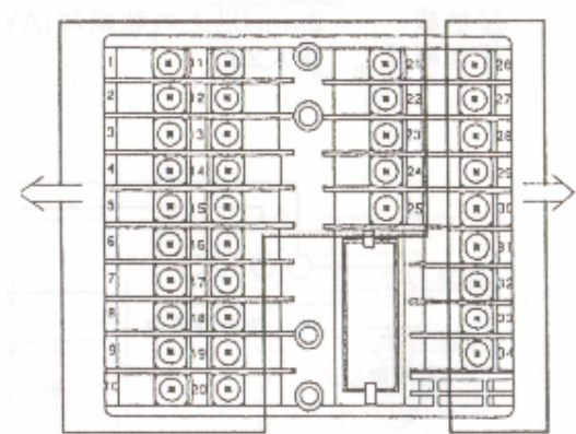
標準端子台
