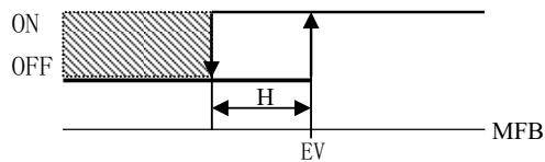
MFB 正
