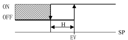
MV 正
