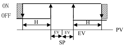
SP 逆
