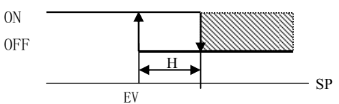
MV 逆
