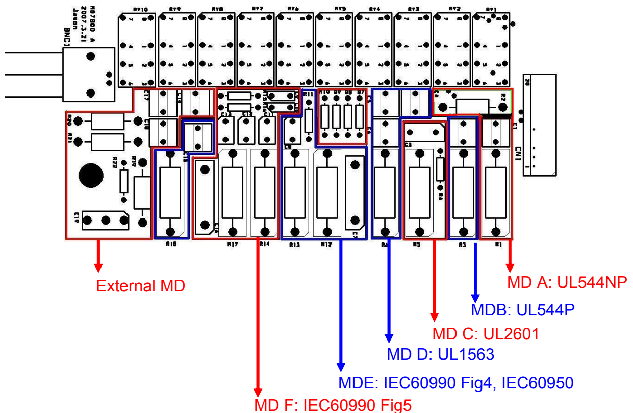
MD 區塊圖
