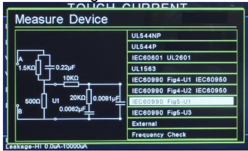
IEC60990 Fig5-U1
