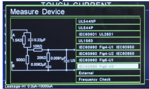
IEC60990 Fig5-U3
