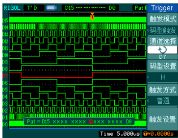
码型触发
