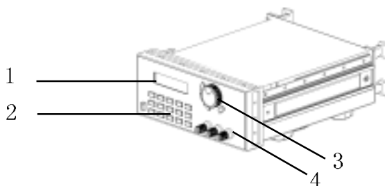
图 1-2 3600 系列电源的面板示意图
