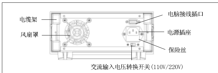
图 1-6 3600 系列电源的背面示意图
