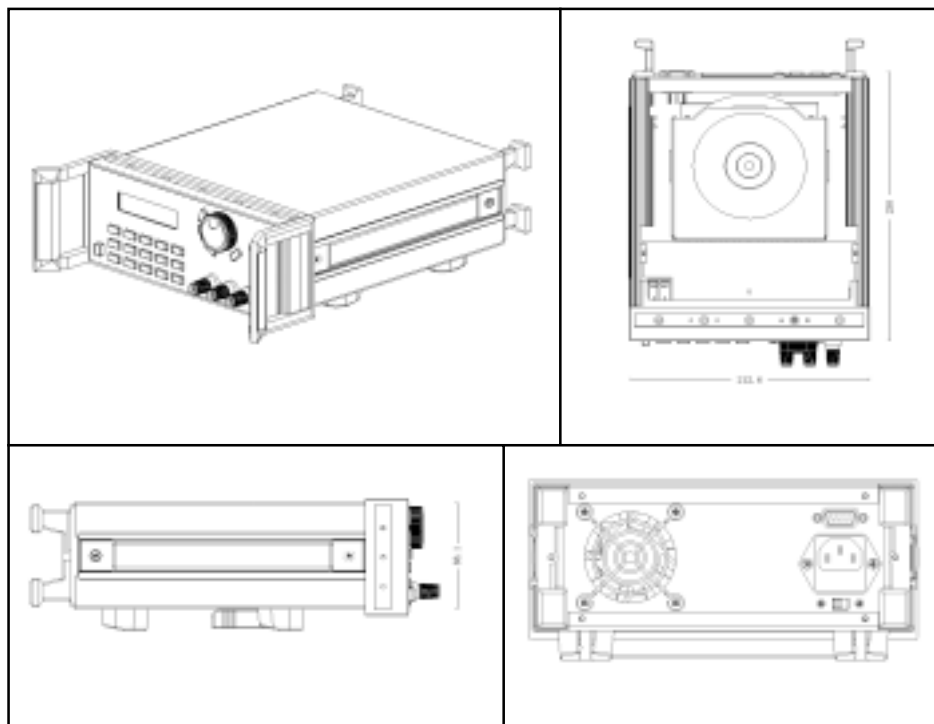
图 1-1 3600 系列可编程直流电源的外观图
