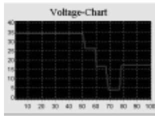
电压运行图
