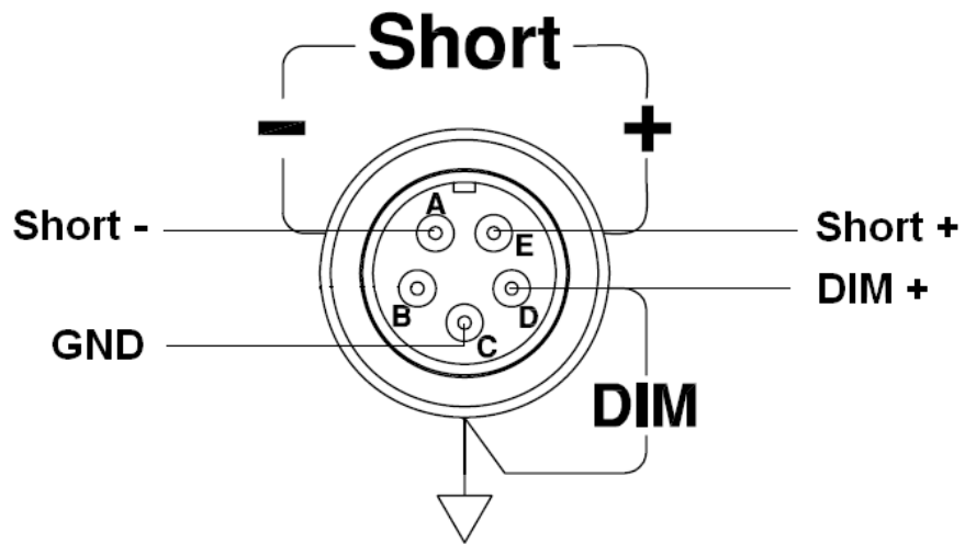
圖 3-4 3340F 系列電子負載Short & DIM 連接方式
