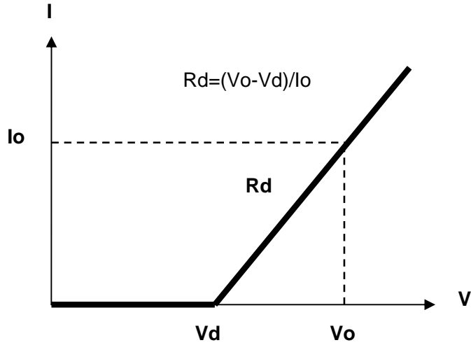
圖 1-8 LED模式特性圖
