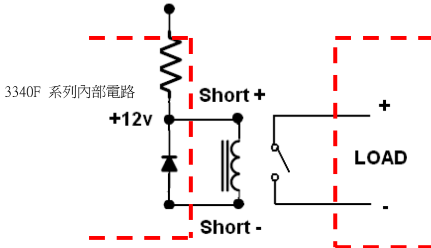
圖4-27 short 測試連接圖
