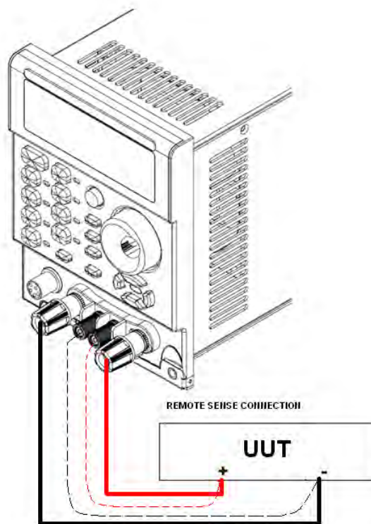
圖 4-2 遠地電壓檢知連接圖
