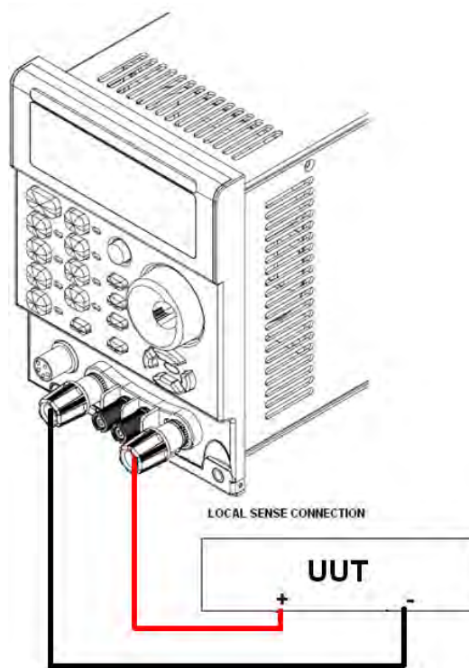
圖 4-1 本地/遠地電壓檢知連接圖
