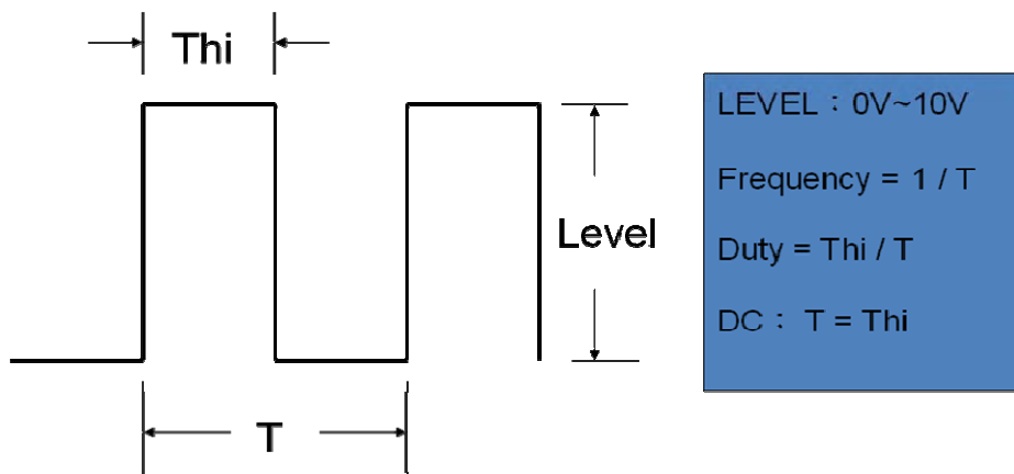
圖 3-3 3340F 系列電子負載 DIM 功能說明
