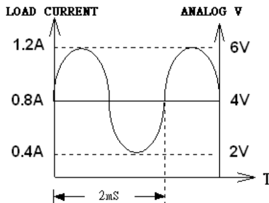
圖 3-5 負載電流之類比設定輸入
