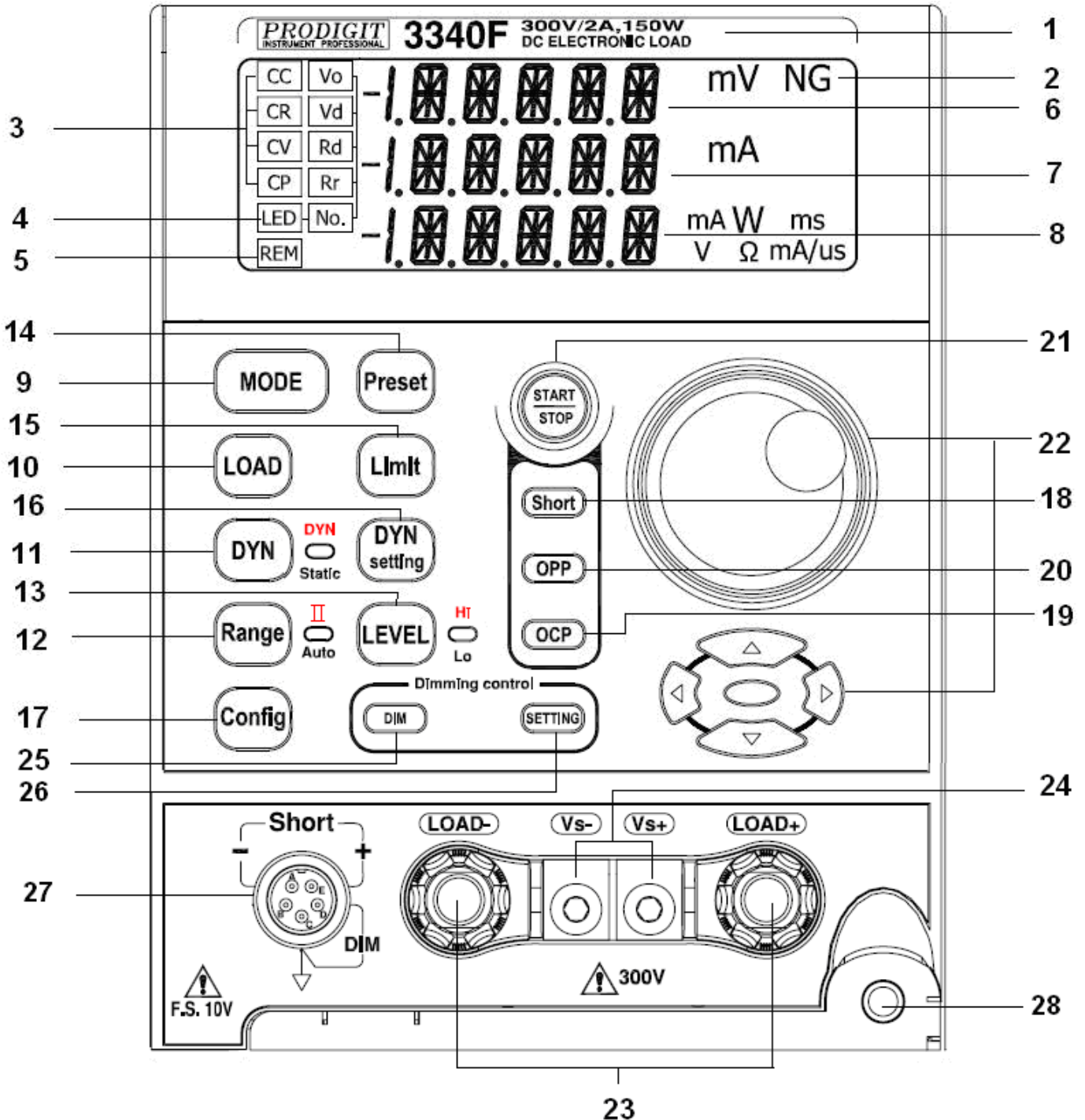
圖 3-1 前面板圖
