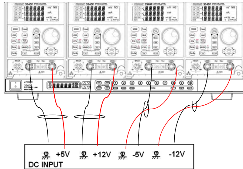
圖 4-23 多組輸出電源供應器與電子負載之連接圖
