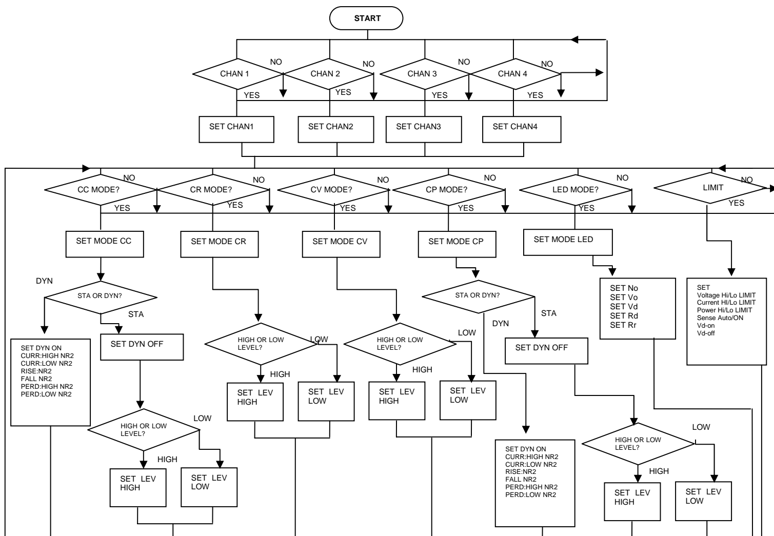
圖 2-3 3340F 系列電子負載操作流程圖
