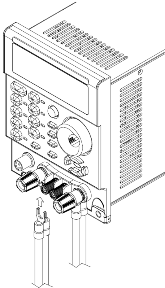
圖3-6 Y型端子連接圖
