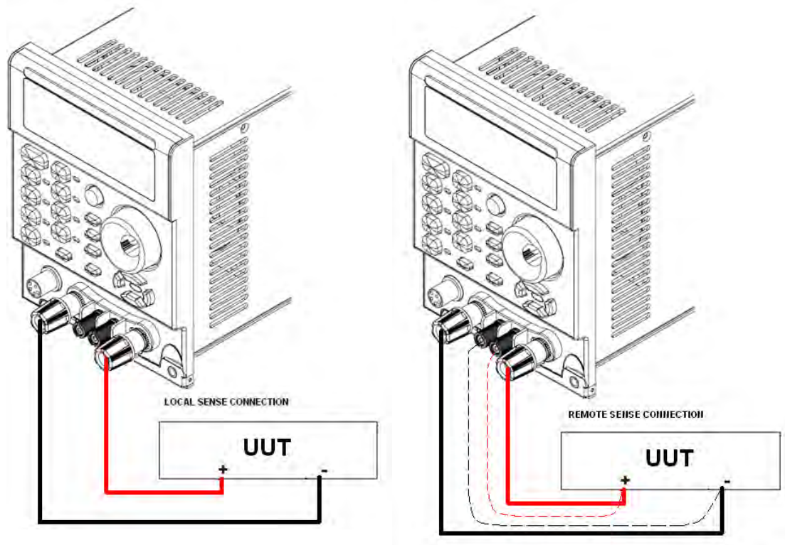
圖 3-2 典型的 3340F 系列電子負載連接方式
