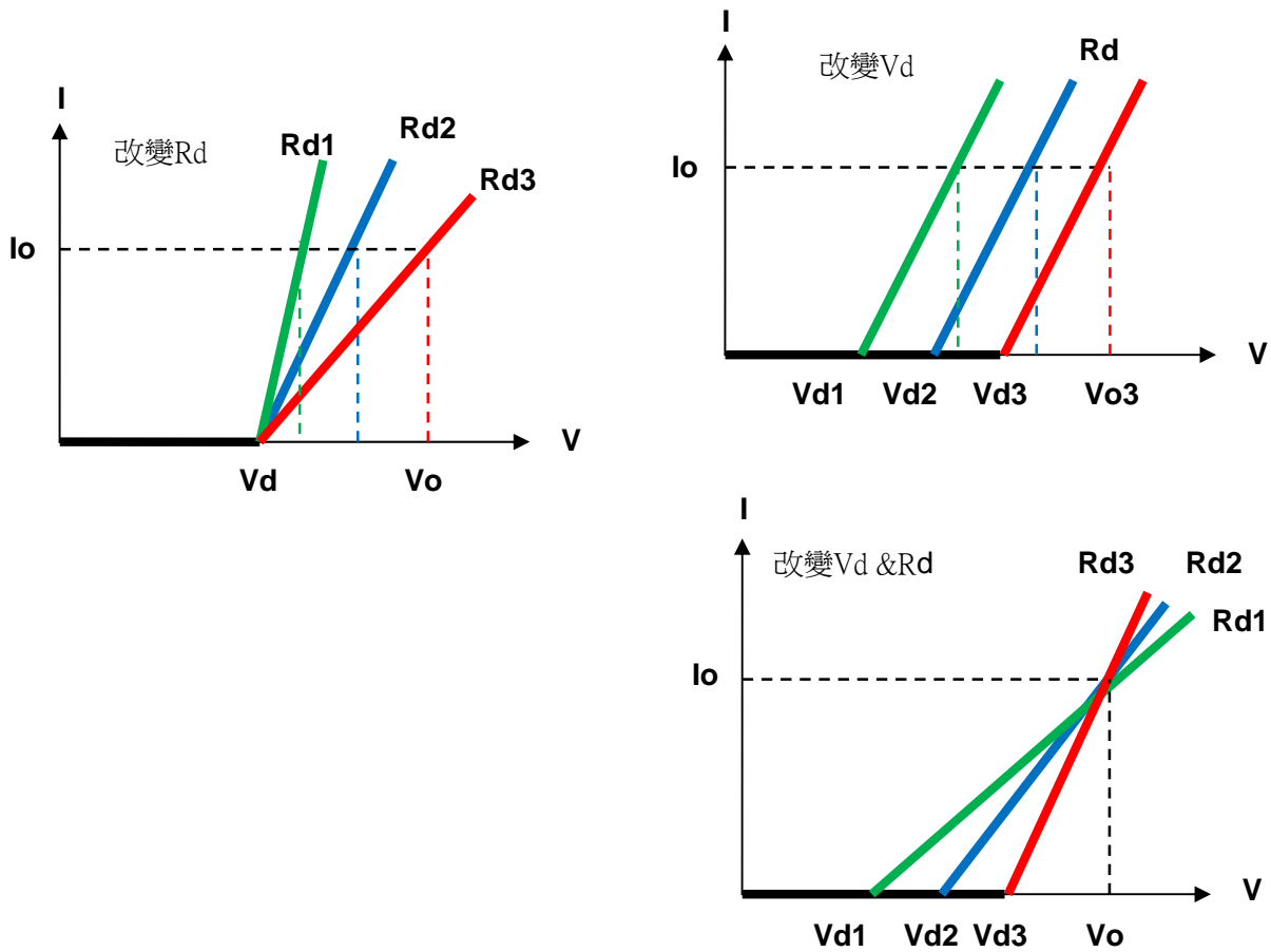
圖 4-21 LED MODE操作模式之應用
