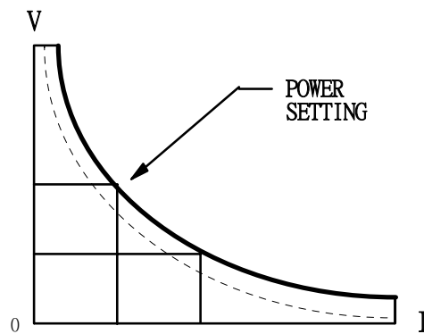
圖 1-7 固定功率模式特性圖
