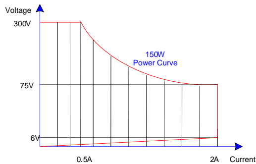
圖 1-1 3340F 0-300V / 0-2A 150W 電子負載功率圖
