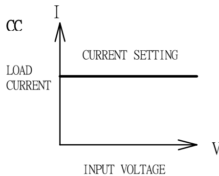
圖 1-4 固定電流模式特性圖
