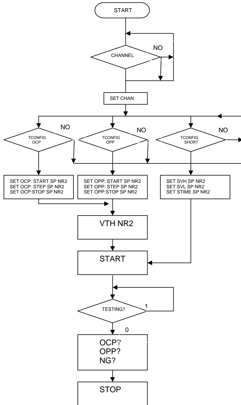
圖 4-26 3340F 系列電子負載OCP、OPP、SHORT操作流程圖
