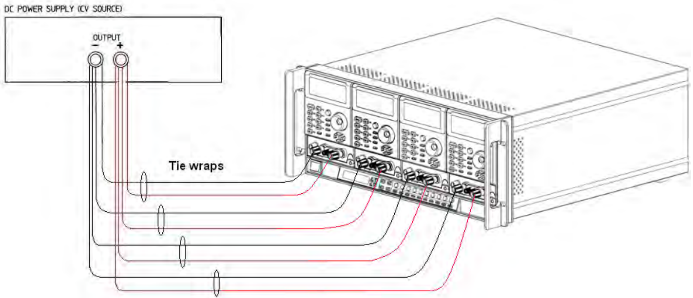
圖 4-24 電子負載多組並聯之連接圖
