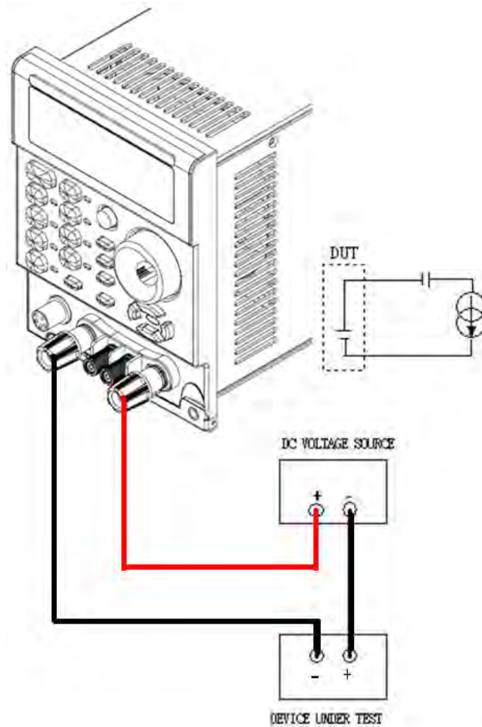
圖 4-25 高功率電子負載最低工作電壓為 0V 時的連接圖
