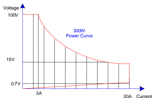
圖 1-2 3341F 0-100V/0-20A 300W 電子負載功率曲線圖
