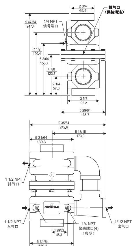
显示有增强密度选项 (L)
