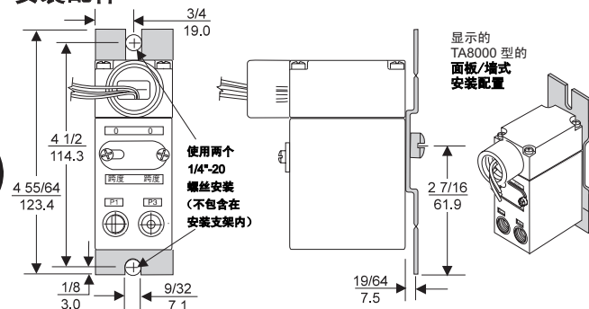
安装支架: 16799-1
