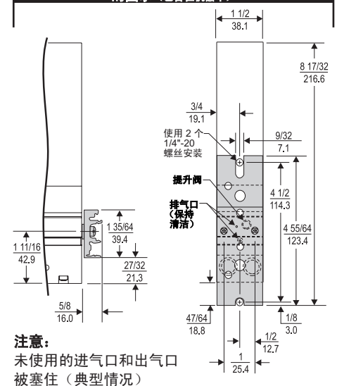
有 DIN 轨道安装配件 16893 和安装配件 16799-1 的图示 (包含在机器中)
