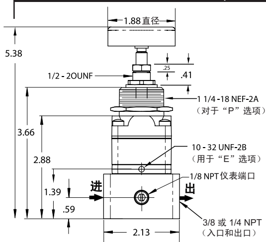
1/4” 和 3/8” NPT 调节器
