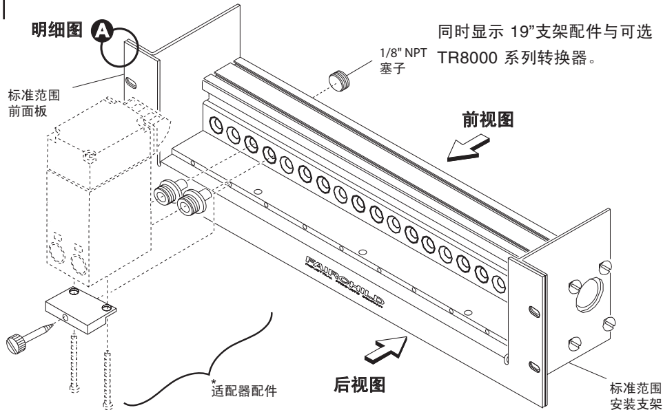
明细图 A — 同时显示标准范围前面板与标准范围安装支架
