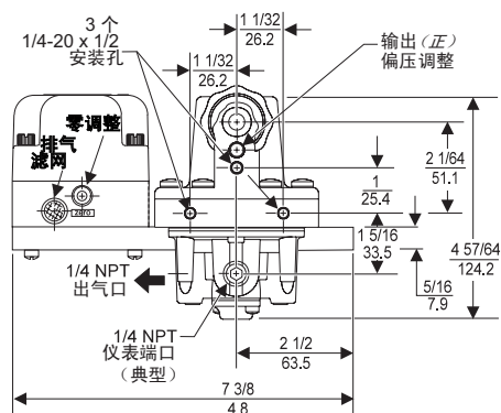
左视图
