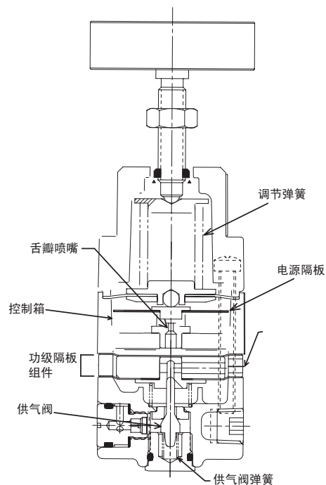
1/8” NPT 调节器
