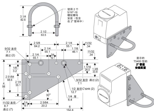
安装支架: 14596
