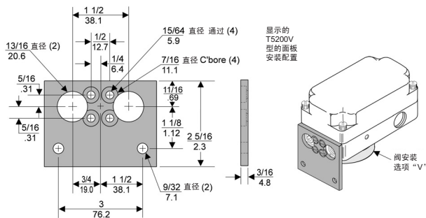
安装支架: 15268
