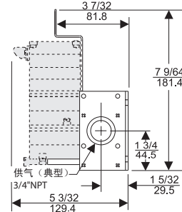
明细图 B — 同时显示标准范围机器和扩展墙式安装支架。
