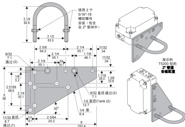
安装支架: 14596
