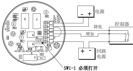
使用隔离双回路电源的控制器（脉冲输入）。
