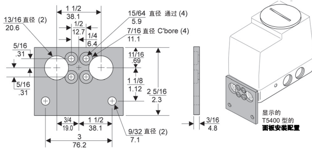
安装支架: 15268
