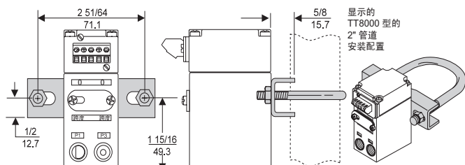
安装支架: 19254-1
