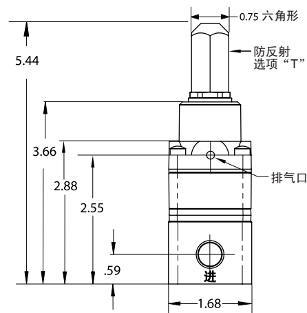
1/4” 和 3/8” NPT 调节器
