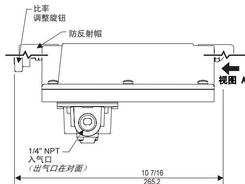
前视图
