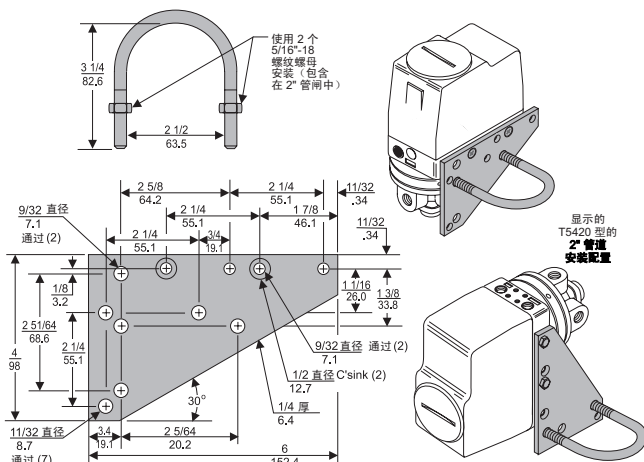
安装支架: 14596
