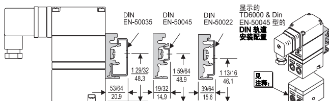
安装支架: 16893-1
