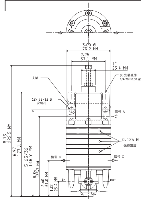
型号: 22112、22113、22212、22213、22222、22223、22312
