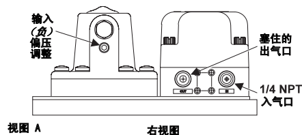
右视图
