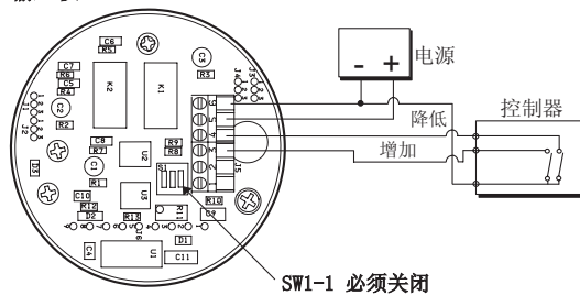
输入板
