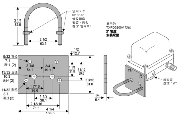
安装支架: 14140
