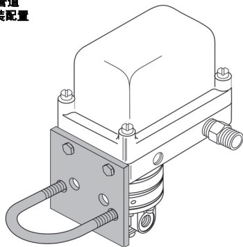
安装配件 14140
