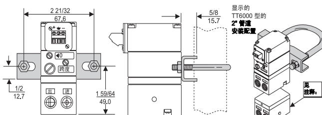
安装支架: 19254-1
