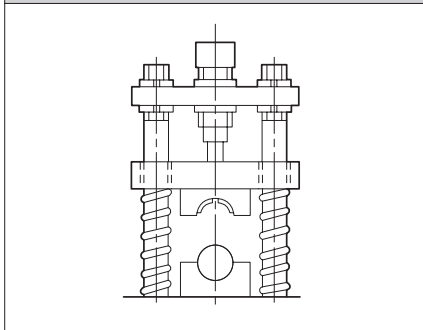
铆接作业
