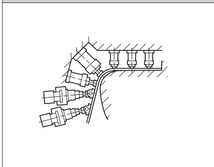
折弯作业
