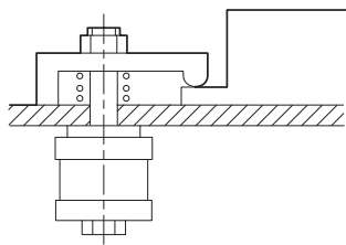
夹紧作业
