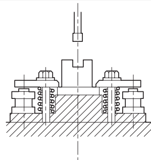
铣削作业
