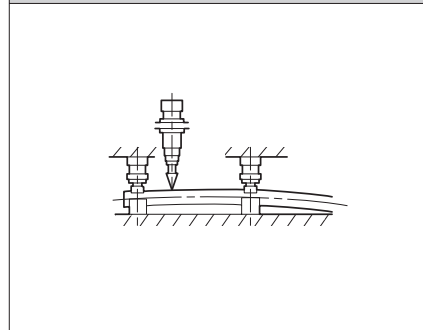
圆棒矫正
