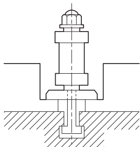
夹紧作业
