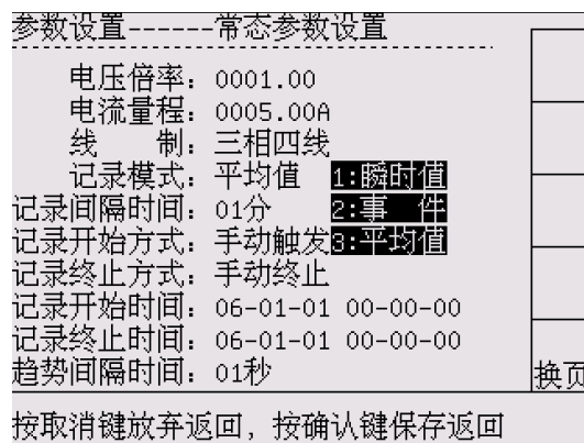
图 5-7 常态设置—记录模式
