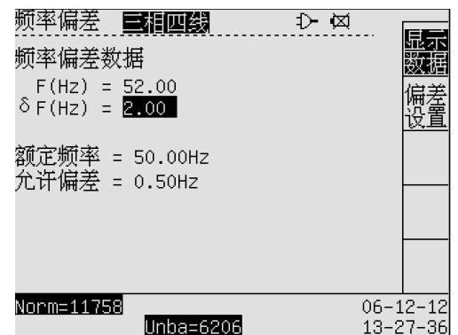
图 10-2 频率偏差屏幕——显示数据
