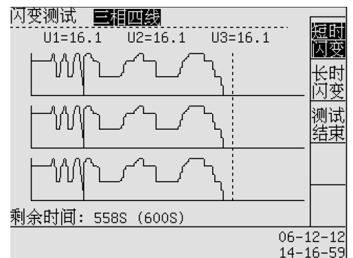
图 12-2 闪变测试屏幕——短时闪变
