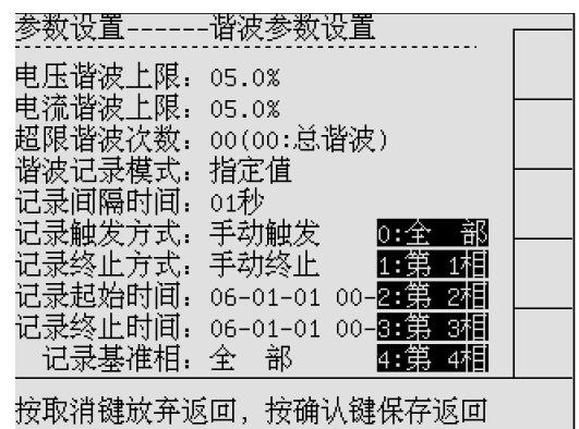
图 11-6 谐波参数—记录基准相
