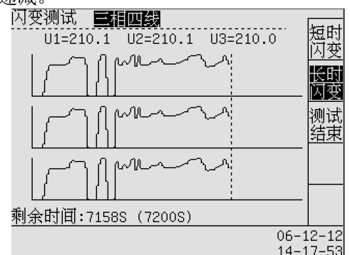
图 12-3 闪变测试屏幕——长时闪变
