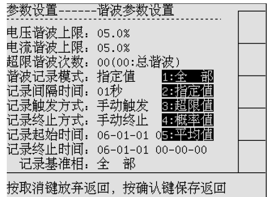
图 11-4 谐波参数—记录模式
