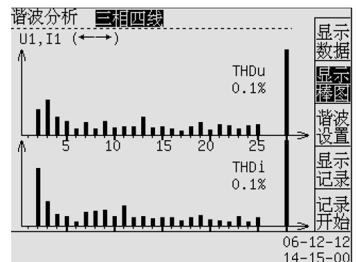
图 11-3 谐波——显示棒图
