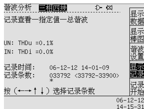
图 11-7 谐波记录
