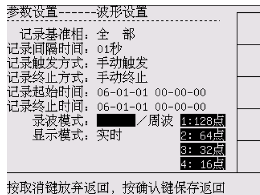
图 6-6 波形设置—录波模式
