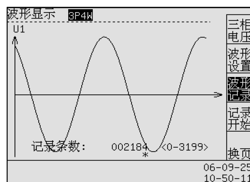
图 6-8 波形记录
