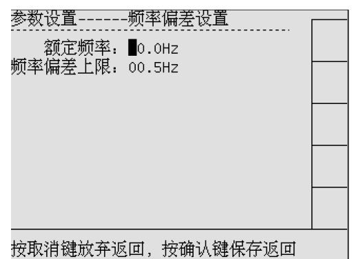
图 10-3 频率偏差屏幕——偏差设置
