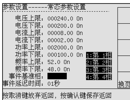
图 5-11 常态设置—事件基准相
