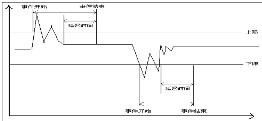
图 5-12 事件描述
