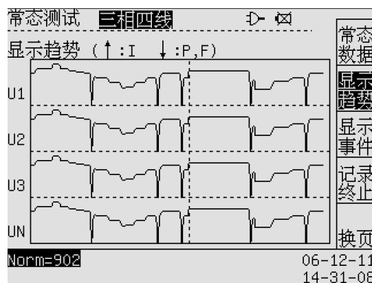
图 5-13 常态—显示趋势
