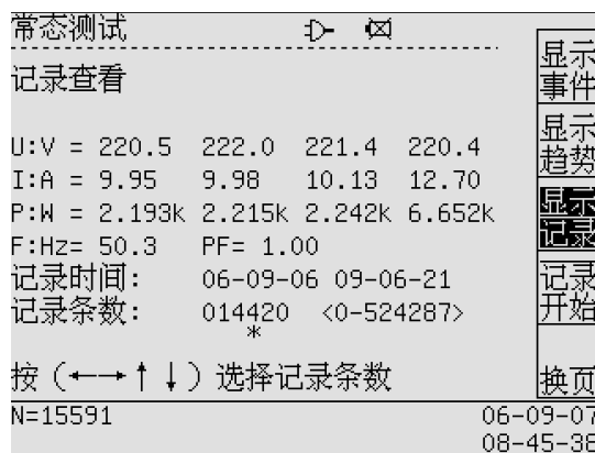
图 5-4 常态记录
