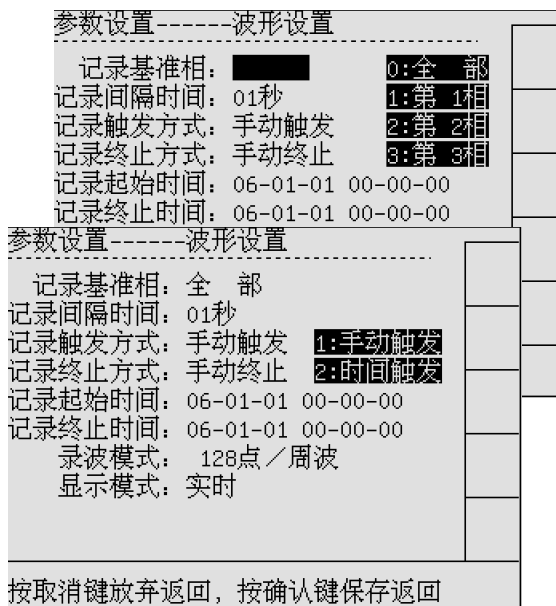
图 6-5 波形设置
