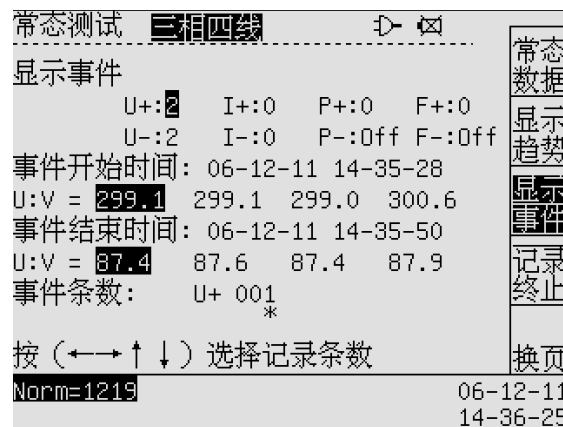
图 5-13 常态—显示事件
