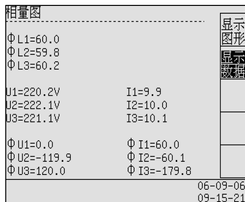
图 7-3 相量图屏幕——显示数据
